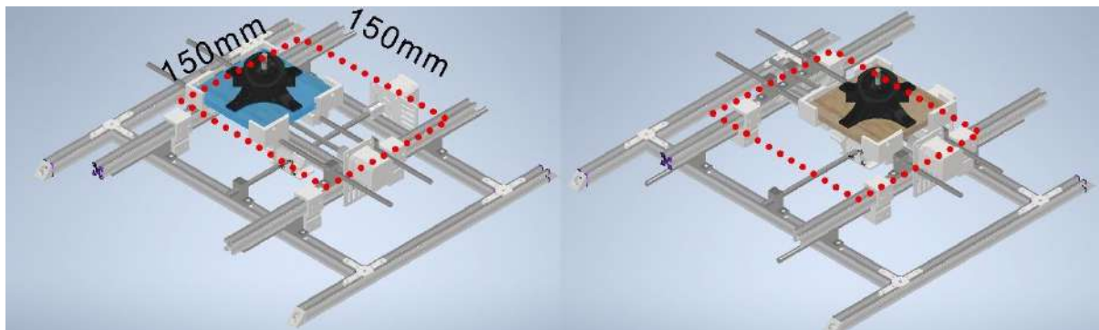
Grafika 14. Wizualizacja zakresu ruchu poziomego podpory ruchomej struktury responsywnej. Skala ruchu dopasowana została do skali struktury. Model komputerowy podpory zrealizowany w programie Autodesk Inventor Professional 2024 stanowi element załącznika nr 5.B pracy.
