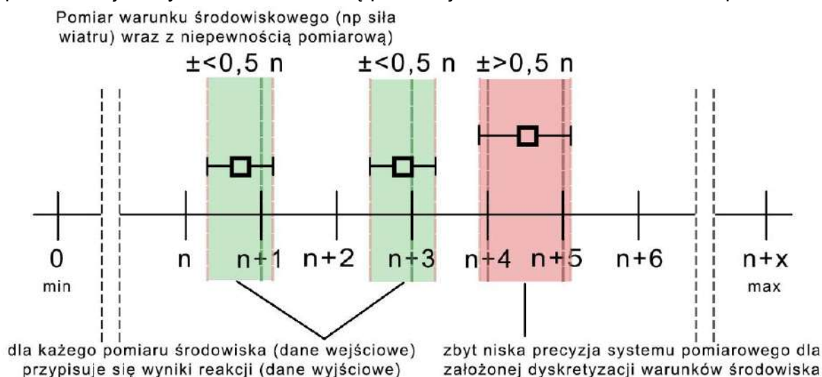
Grafika 3. Schemat przedstawia wpływ dokładności pomiarów na skuteczność reakcji systemu. Gdy pomiary nie zachowują odpowiedniej precyzji następuje błędne rozpoznanie przypadku obciążeniowego. W konsekwencji występuje możliwość przeciążenia struktury.
