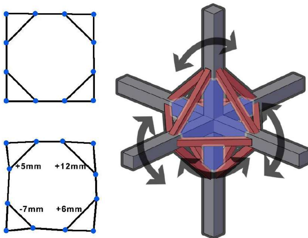
Grafika 46. Schemat strefy węzłowej struktury ramowej. Grafika przedstawia złożoność sterowania każdym z elementów modelu. Ruch wykonywany jest w 3 płaszczyznach dla wszystkich belek oraz słupów.
