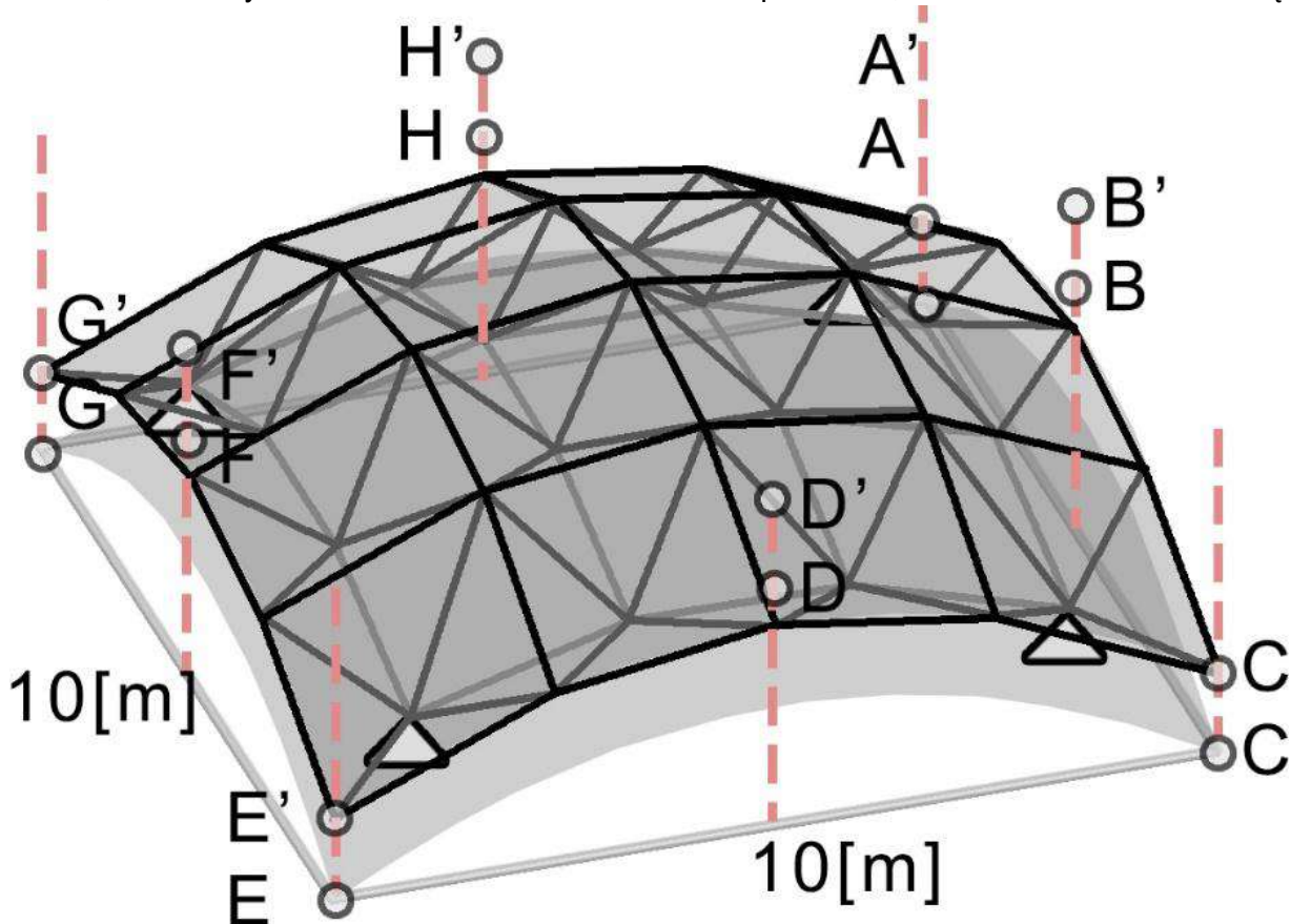
Grafika 8. Schemat budowy modelu komputerowego kratownicy przestrzennej wraz z punktami kontrolnymi umożliwiającymi sterowanie modelem
