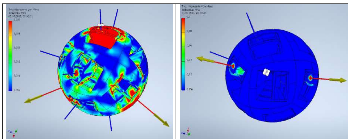
Grafika 92. Wyniki graficzne analizy MES modelu węzła centrycznego. Na lewej grafice przedstawiono wyniki ze sztucznym ograniczeniem zakresu do 5kPa, natomiast z prawej strony przedstawiono nieskalowany wykres graficzny naprężeń dochodzący do 0,1MPa.
