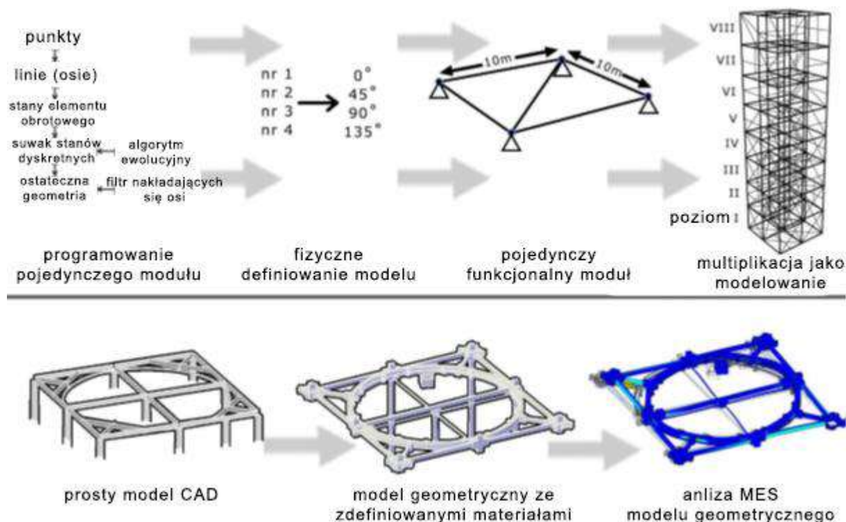
Grafika 99. Zaprogramowanie modelu badawczego opierało się na połączeniu szeregu powtarzanych modułów w jednolitą strukturę. Osobno prowadzono badania zachowania całego modelu oraz pojedynczego modułu uwzględniającego geometryczną złożoność koncepcji.
