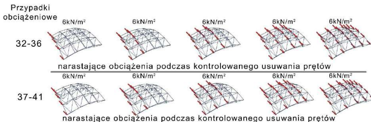
Grafika 62. Zestawienie przypadków obciążeniowych dla modeli preakcji. Wszystkie przypadki symulowane są grupami obciążeń punktowych lub obciążeniami powierzchniowymi o stałym charakterze oddziaływania.
