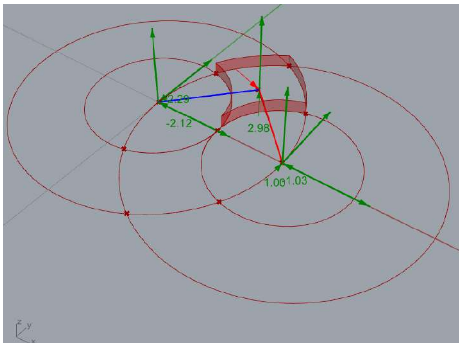
Grafika 22. Przedstawienie aksonometryczne zakresu przestrzeni ruchu podpory powłoki.
