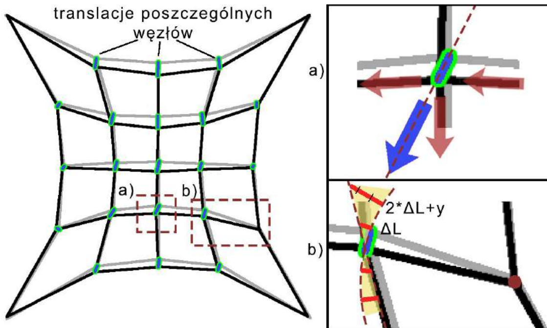
Grafika 72. Schematyczne przedstawienie złożoności ruchu modelu kratownicy, w którym wszystkie elementy nośne pozostają ruchome. Teoria ruchu i nieliniowej pracy siłowników.
