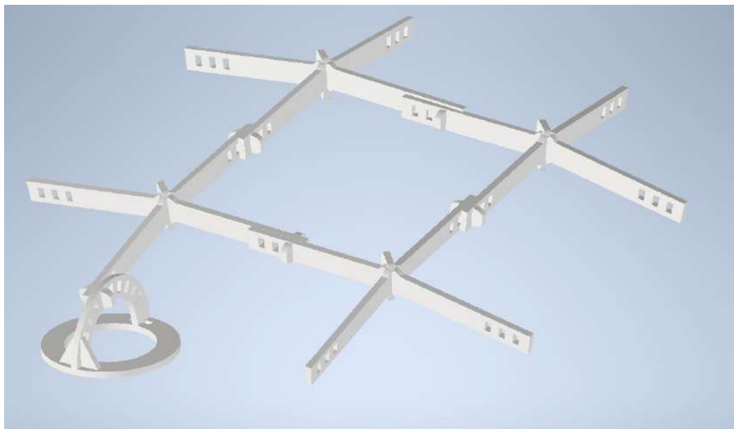
Grafika 30. Przedstawienie modularnego systemu elementów łączników tworzących szalunki dla deformacji płaskiej płyty poliwęglanowej. Model opracowany w programie Autodesk Inventor Professional i stanowi załącznik nr pracy.
