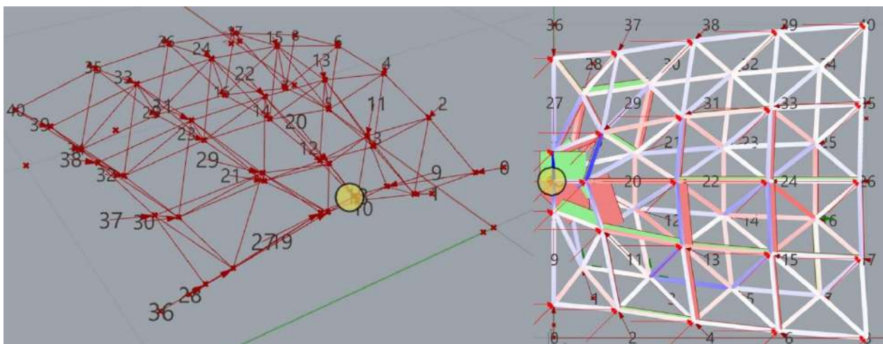
Grafika 65. Przykładowy wynik deformacji geometrii kratownicy przez model nr 2 wraz z prezentacją wykresów naprężeń dla poszczególnych prętów. Zauważalne są główne kierunki przenoszenia naprężeń w stronę wszystkich podpór modelu. Im bardziej linia łącząca punkt przyłożenia siły z podporą pokrywała się z układem prętów, tym większy wzrost efektywności model wykazywał.
