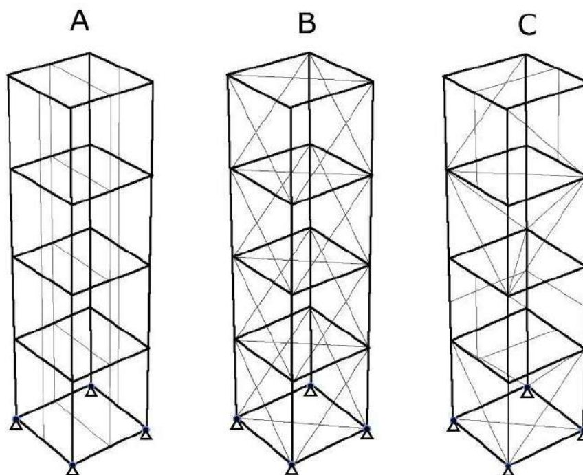
Grafika 101. Trzy kolejne układy skratowań modeli złożonych z modułów responsywnych topologicznie. Model "A" jest bazowym układem nie optymalizowanym pod względem strukturalnym. Układ "B" stanowi proste skratowanie efektywne, powszechnie stosowane szczególnie przy użyciu cięgien. Model „c” stanowi przykładowe skratowanie sterowane algorytmem ewolucyjnym.
