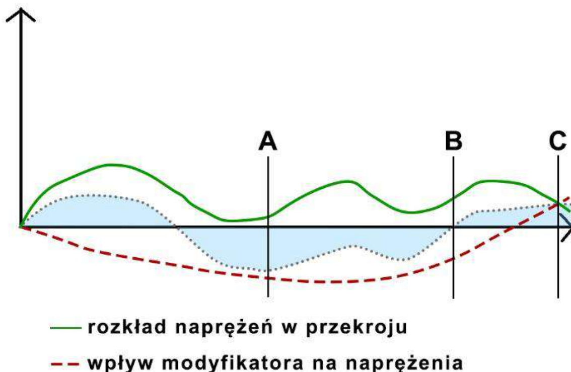
Grafika 42. Interpolacja wyników naprężeń z różnych źródeł oraz interpretacja wartości dla różnych przypadków geometrycznych.
