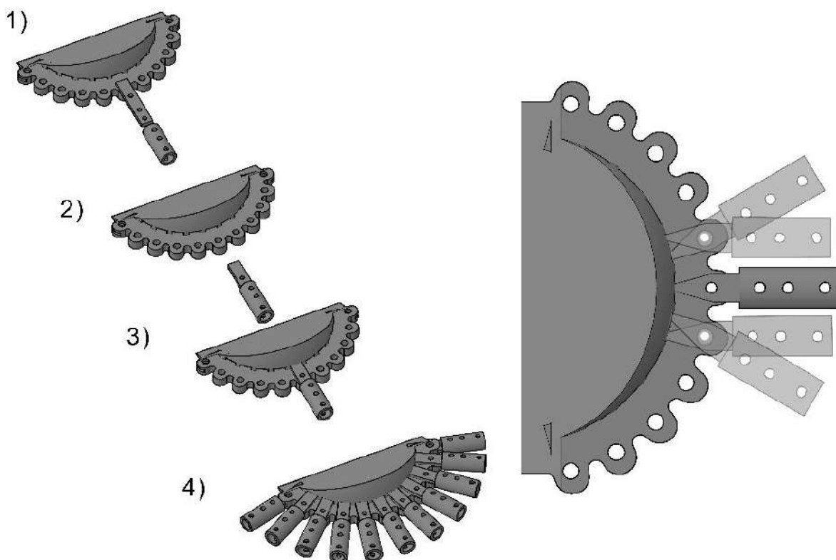
Grafika 83. Sposób łączenia pręta z elementem węzłowym. Na prawej grafice widoczny jest zakres rotacji każdego z prętów pozwalający na ruch modelu responsywnego.
