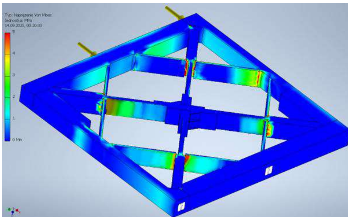
Grafika 114. Wyniki analizy MES pojedynczego modułu responsywnego topologicznie. Widoczne są wzrosty naprężeń na elementach 3 fazy rozkładania.
