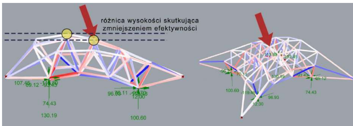
Grafika 66. Przykładowy wynik geometrycznej modyfikacji kratownicy wraz z przedstawionym problemem skali reakcji wpływającym na nieefektywną proporcję wysokości poszczególnych węzłów modelu.
