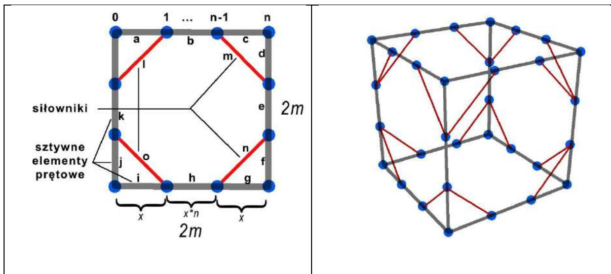
Grafika 44. Koncepcja modularnej struktury modyfikatorów oraz sposobu sterowania zmianami geometrii struktur sztywnych węzłowo.
