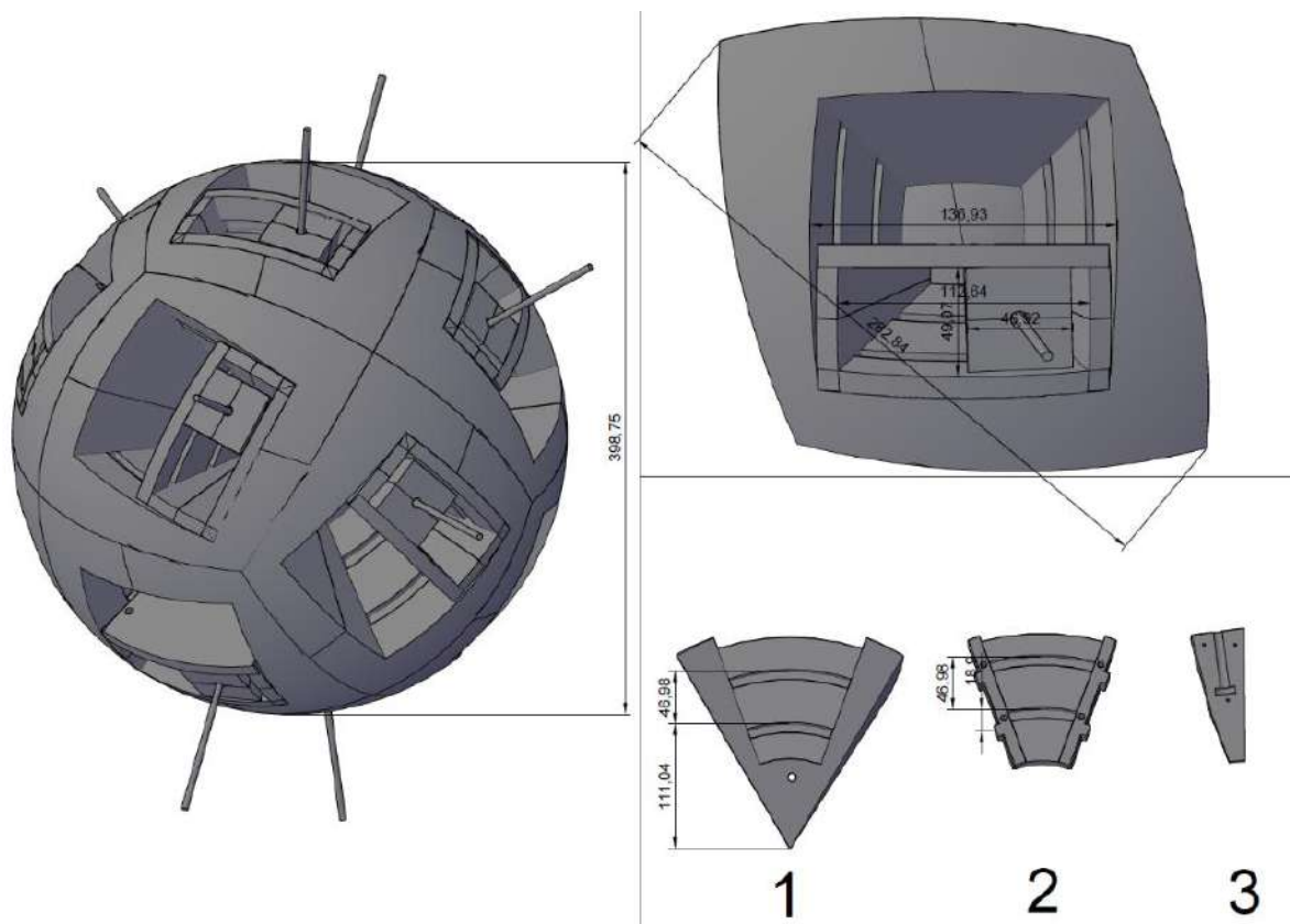
Grafika 90. Koncepcja modelu węzła centrycznego z przedstawieniem elementów składowych powtarzalnej struktury dwunastościanu.
