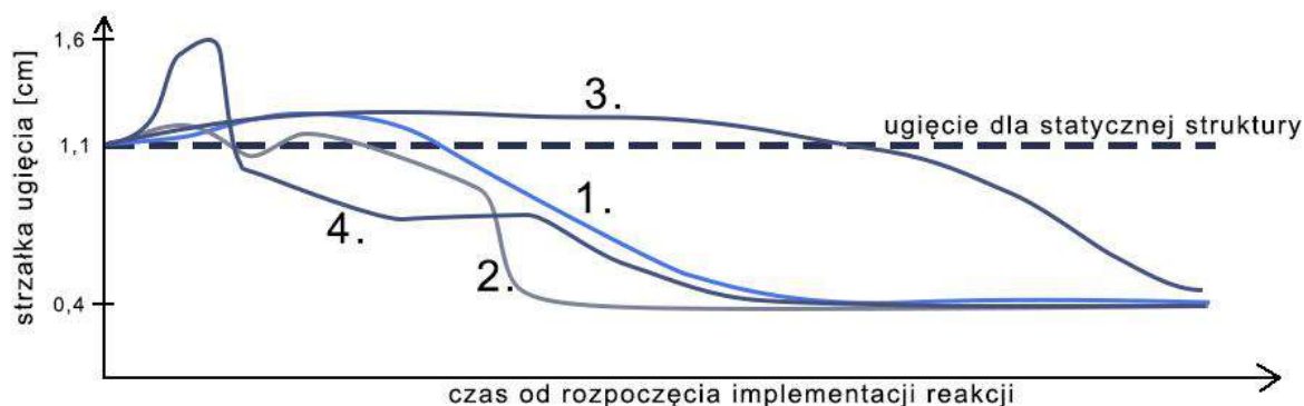
Grafika 68. Wykresy zmian wartości ugięć podczas ruchów pośrednich dla wszystkich modeli. Zauważalne jest, że wszystkie modele przekraczają chwilowo maksymalne naprężenia referencyjnej struktury statycznej.
