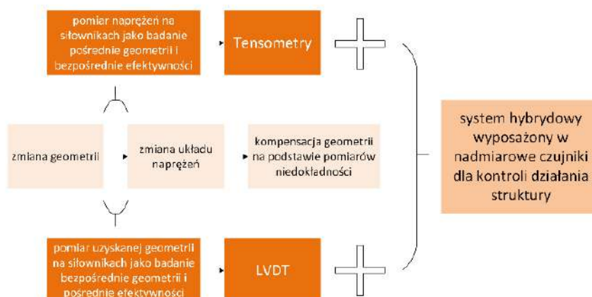
Grafika 4. Schemat blokowy dwóch systemów koniecznych do wprowadzenia w strukturze responsywnej. Systemy te podlegają coraz częściej unifikacji w jeden kompleksowy system..
