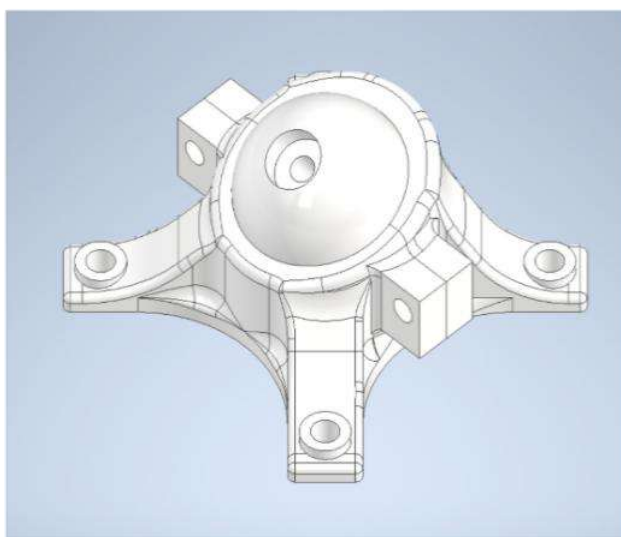
Grafika 85. Przedstawienie sposobu uzyskania rotacji na węźle. PO prawej stronie widoczna forma bryły, na której oparta została koncepcja modelu bryłowego węzła dla struktur responsywnych.
