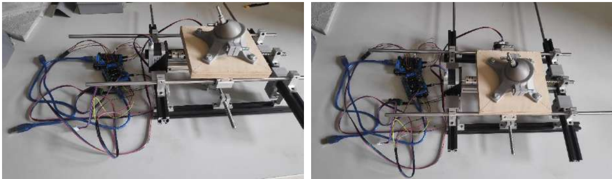
Grafika 18. Gotowy fizyczny model struktury responsywnej, w pełni funkcjonalny, umożliwiający do przesuwu przy siłach poziomych do 200N.
