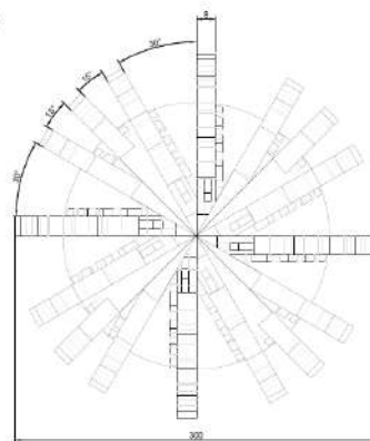
moduł międzypasmowy 3-gniazdowy
