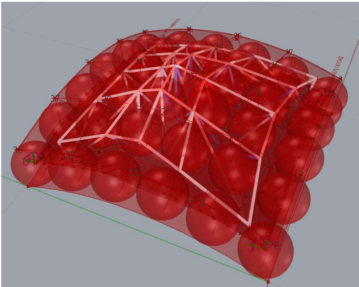
Grafika 60. Przykład geometrii kratownicy uzyskany w wyniku działania modelu opartego o koncepcję strumieni sił. Każda ze sfer reprezentuje zakres wpływu strumieni na poszczególne węzły.
