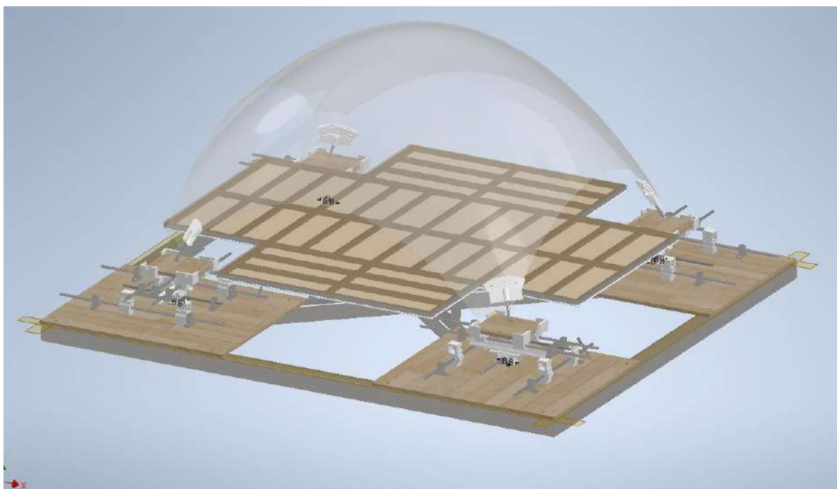
Grafika 29. Widok aksonometryczny koncepcji modelu fizycznego ruchomej powłoki wykorzystującej zjawisko elastooptyczne do wizualizacji naprężeń.
