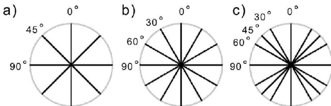
Grafika 82. Koncepcja modelowania ramion połączeń węzła ze względu na dostępność uzyskiwanych geometrii struktur przestrzennych i minimalizację nieosiowości.
