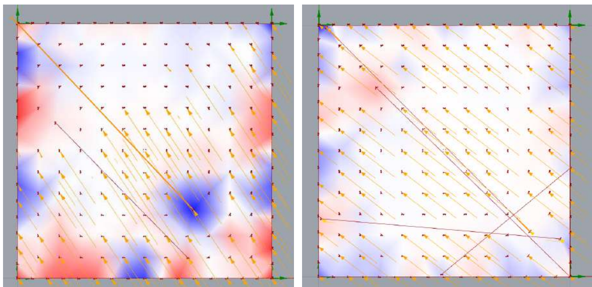
Grafika 40. Tendencje modyfikatorów do uzyskiwania układów analogicznych do ściągów struktur powłokowych w celu redukcji sił poziomych w modelu. Układy takie ze względu na znaczne długości modyfikatorów uzyskują bardzo nieefektywne topologie.
