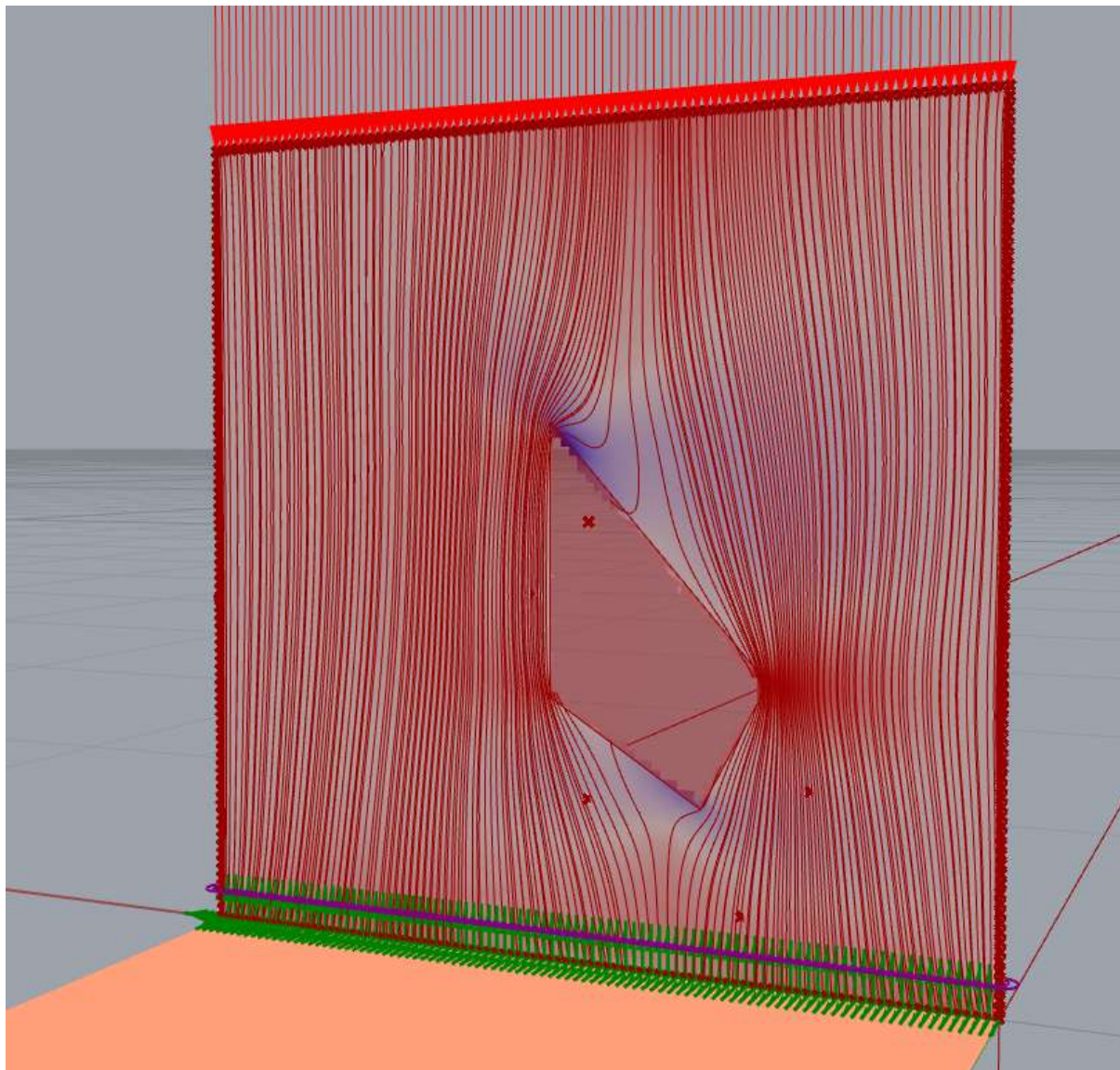
Grafika 59. Przykładowy wykres strumieni sił według teorii rozkładu naprężeń według prof. Wacława Zalewskiego. Widoczny jest wpływ naroży otworowań na rozkład strumieni. Układ strumieni sił jest komplementarny z mapą naprężeń. W miejscu zwiększonego zagęszczenia linii strumieni mapa przyjmuje wyraźniejszy kolor sygnalizując większe naprężenia.
