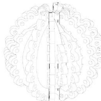
Grafika 84. Ostateczna koncepcja modelu elementów węzłowych pozwalających na uzyskanie wystarczającego stopnia obrotu wszystkich elementów ruchomych względem elementów statycznych.
