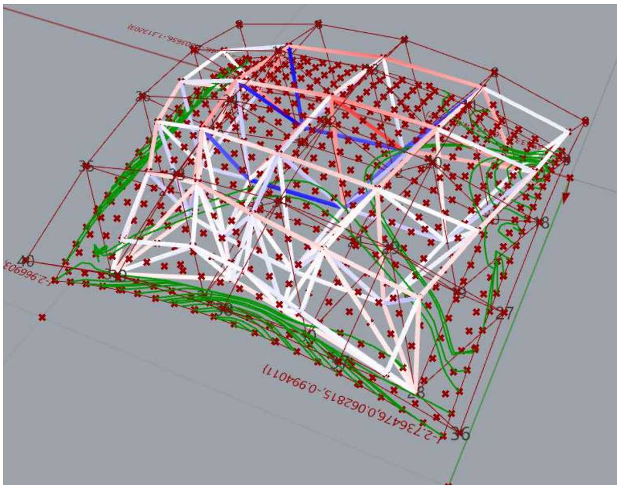
Grafika 67. Rozkład strumieni sił na referencyjnym modelu powłoki. Na jego podstawie obliczana jest deformacja kratownicy. Wynik deformacji przedstawiony jest wraz z graficznym wynikiem rozkładu naprężeń na grafice.
