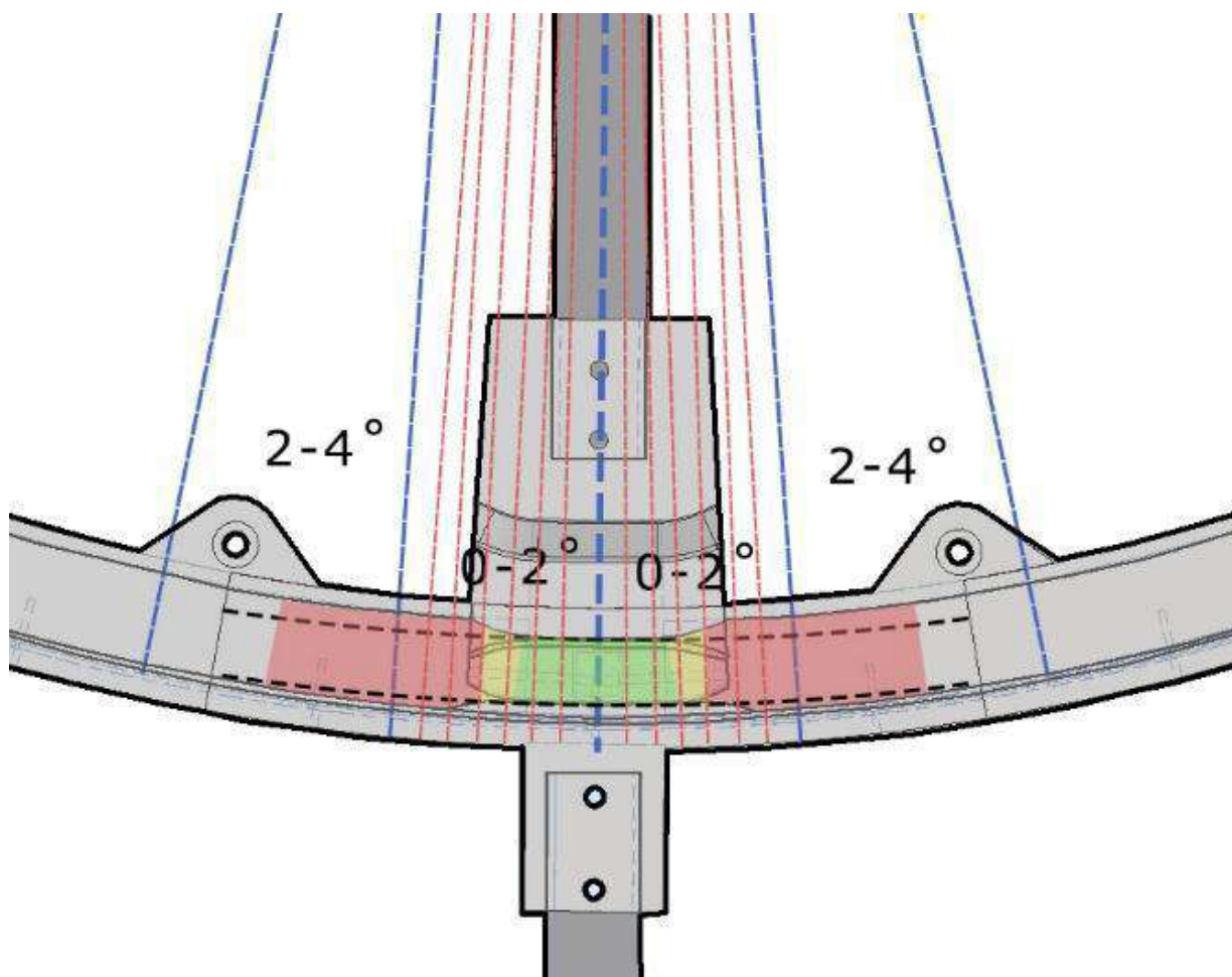
Grafika 109. Strefy wpływu niedokładności połączeń na rozkład naprężeń. Zaznaczono na podstawie wyników zakresy poprawne, dopuszczalne oraz niepoprawne pozycjonowania belki. Zakres pozostaje indywidualny dla zamodelowanej geometrii elementów oraz całego modułu.
