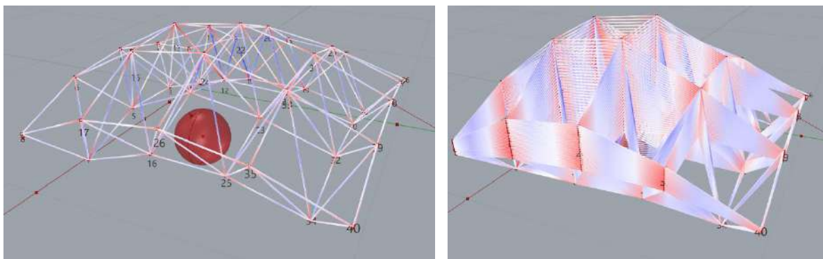
Grafika 56. Schemat działania modelu zwiększania grubości kratownicy. Na grafice prawej widocznych jest wszystkie 50 geometrii badanych jednocześnie. Model stanowi załącznik nr 8.b pracy.
