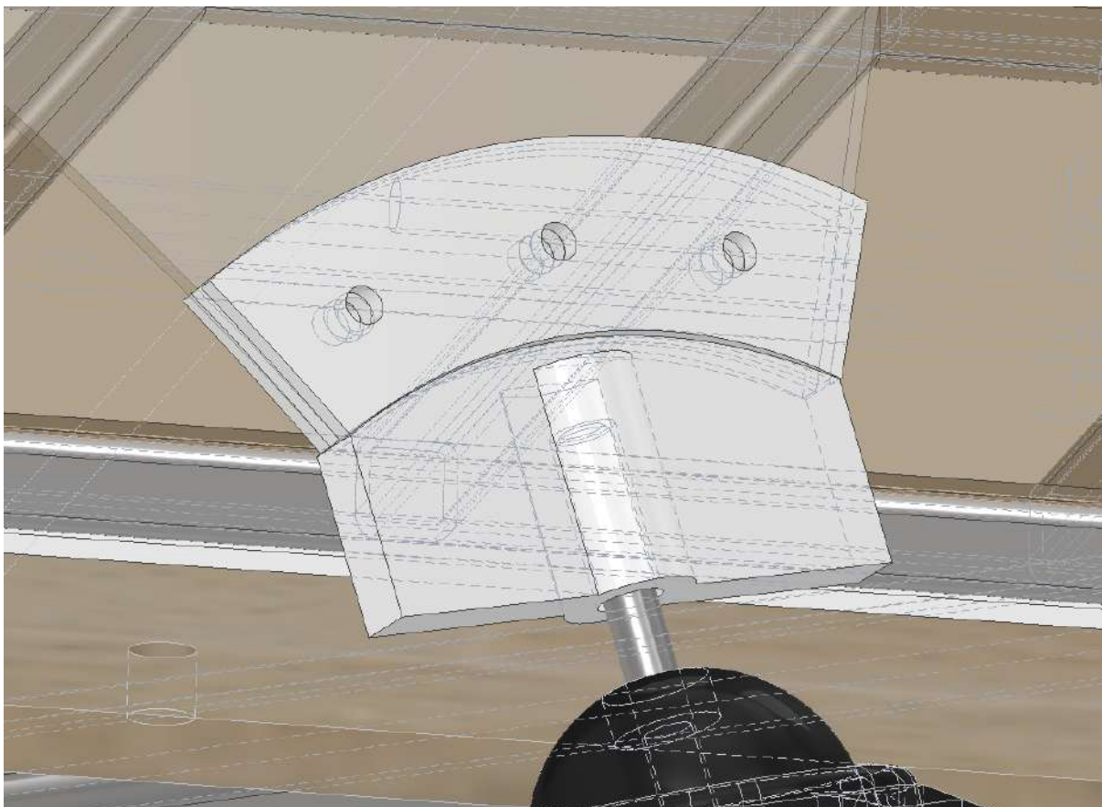
Grafika 20. Przedstawienie modelu mocowania powłoki do podpory. Pozwala ono na jednorodną dystrybucję naprężeń między elementami oraz uniknięcie zmiany znaku naprężeń w narożu modelu.
