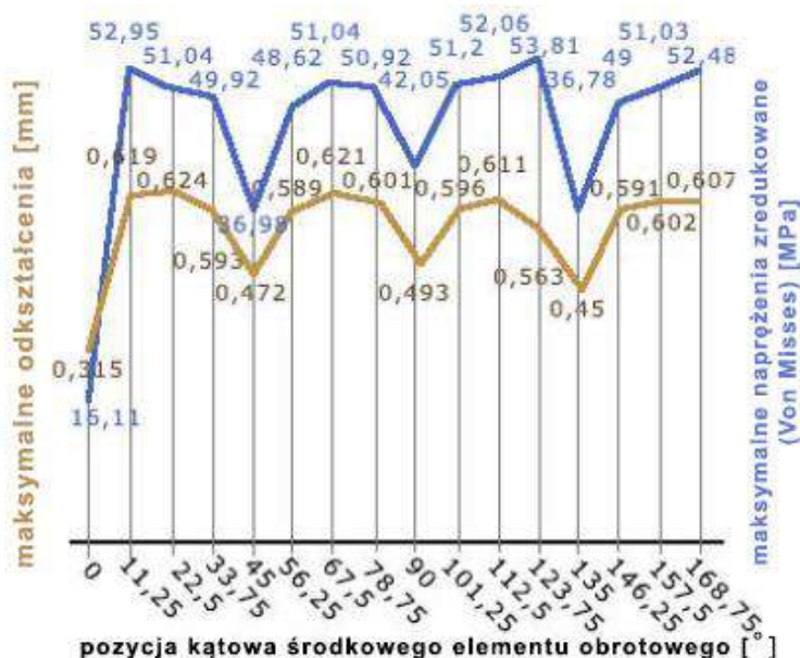
Grafika 107. Wykres wartości dyskretnych ugięć oraz naprężeń dla poszczególnych pozycji belki środkowej oznaczonych przez określenie jej kąta względem pozycji referencyjnej dla pojedynczego przypadku obciążeniowego.
