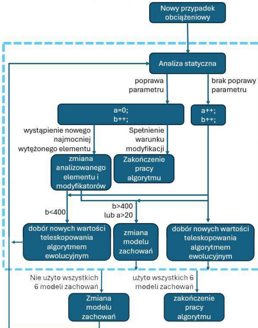
Grafika 53. Schemat działania modelu zachowań hybrydowo-iteracyjnego pozwalającego na przyspieszenie reakcji struktury.
