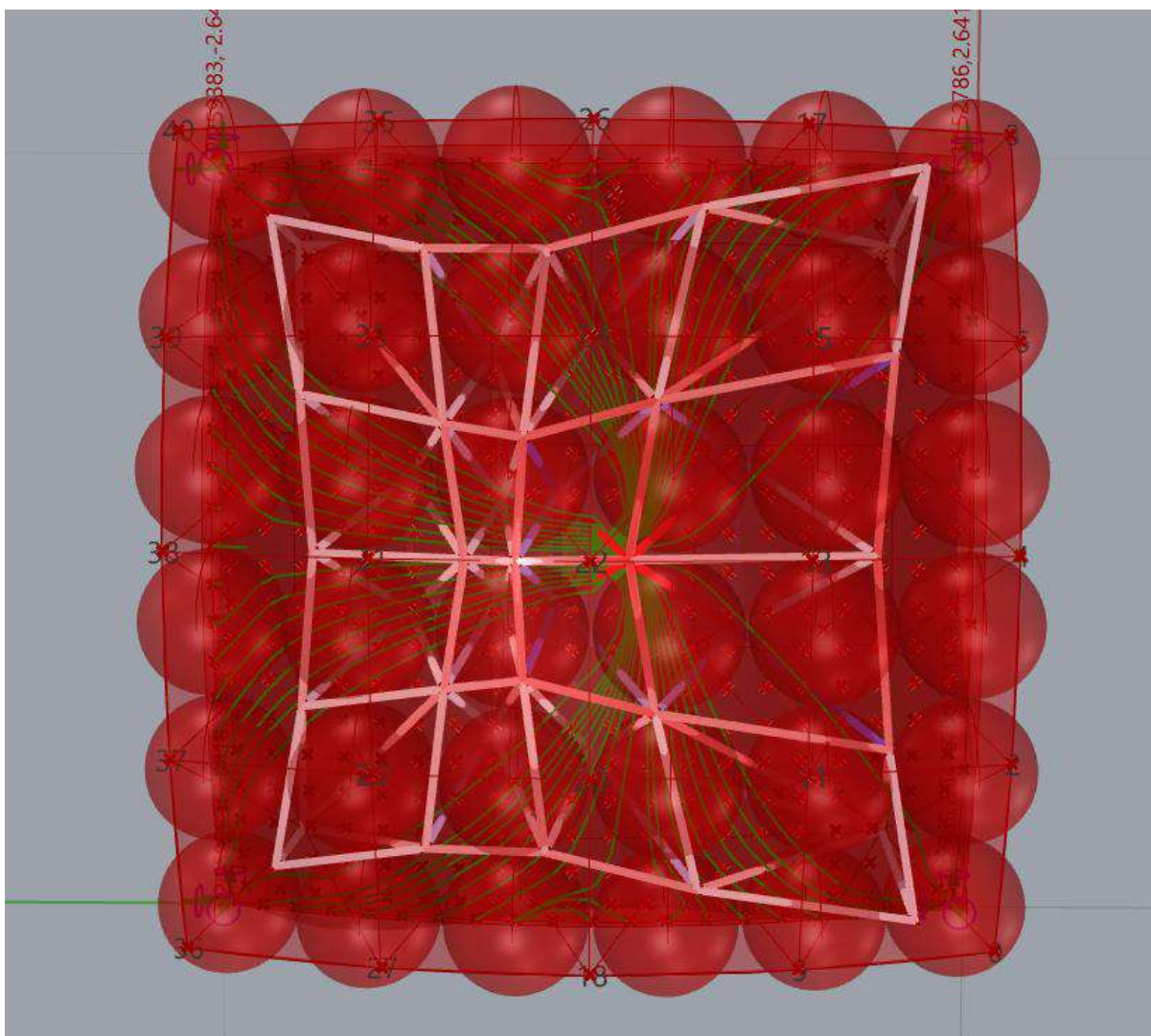
Grafika 61. Układ geometryczny w widoku z góry. Zauważalny jest największy wpływ węzłów środkowych na geometrię kratownicy referencyjnej. Model stanowi załącznik nr 8.C pracy.
