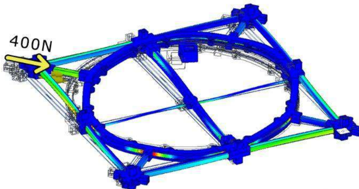
Grafika 108. Przypadek obciążeniowy dla którego przeprowadzano badania pozycji dyskretnych. Dla każdego przypadku przeprowadzano analizę z użyciem MES i generowano wyniki w postaci mapy naprężeń.
