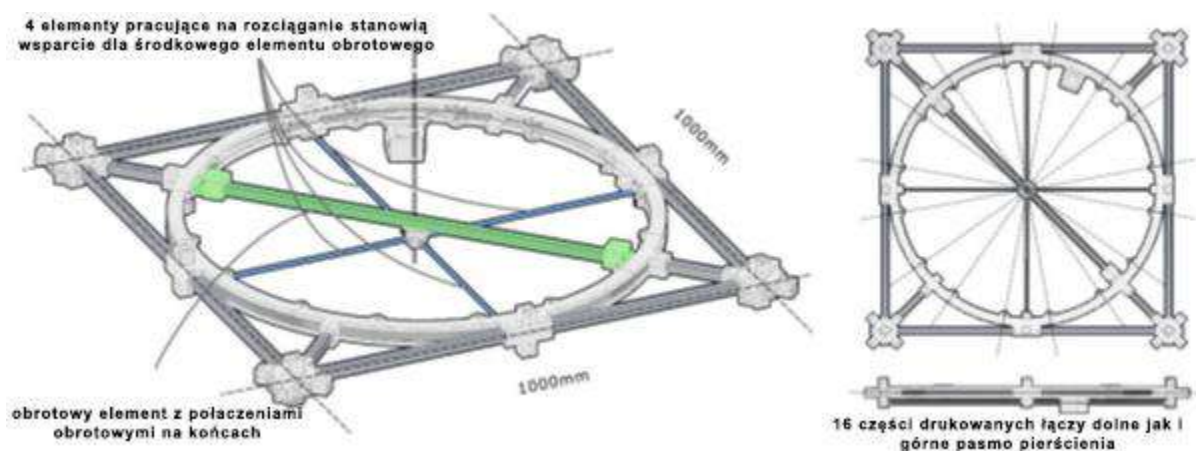
Grafika 106. Koncepcja modelu modułu powtarzalnego responsywnego topologicznie opracowanego na podstawie teorii ruchu opisanej we stępie badań. Struktura dzieli się na część ruchomą oraz statyczną. Zachowuje sztywność nawet przy usunięciu elementu ruchomego, lecz przy jego użyciu podnosi parametry statyczne struktury
