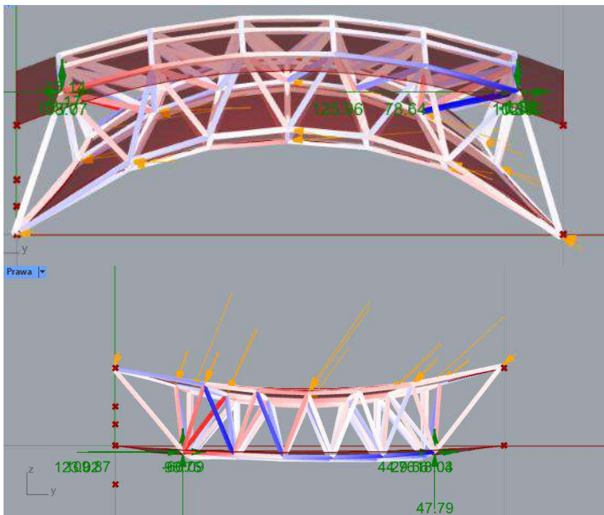
Grafika 80. Wynik modyfikacji geometrii fragmentów struktury. Zauważalna jest różnica proporcji reakcji geometrycznych systemu. Dolne pasmo wymaga ruchu o znacznie większej skali niż pasmo górne.
