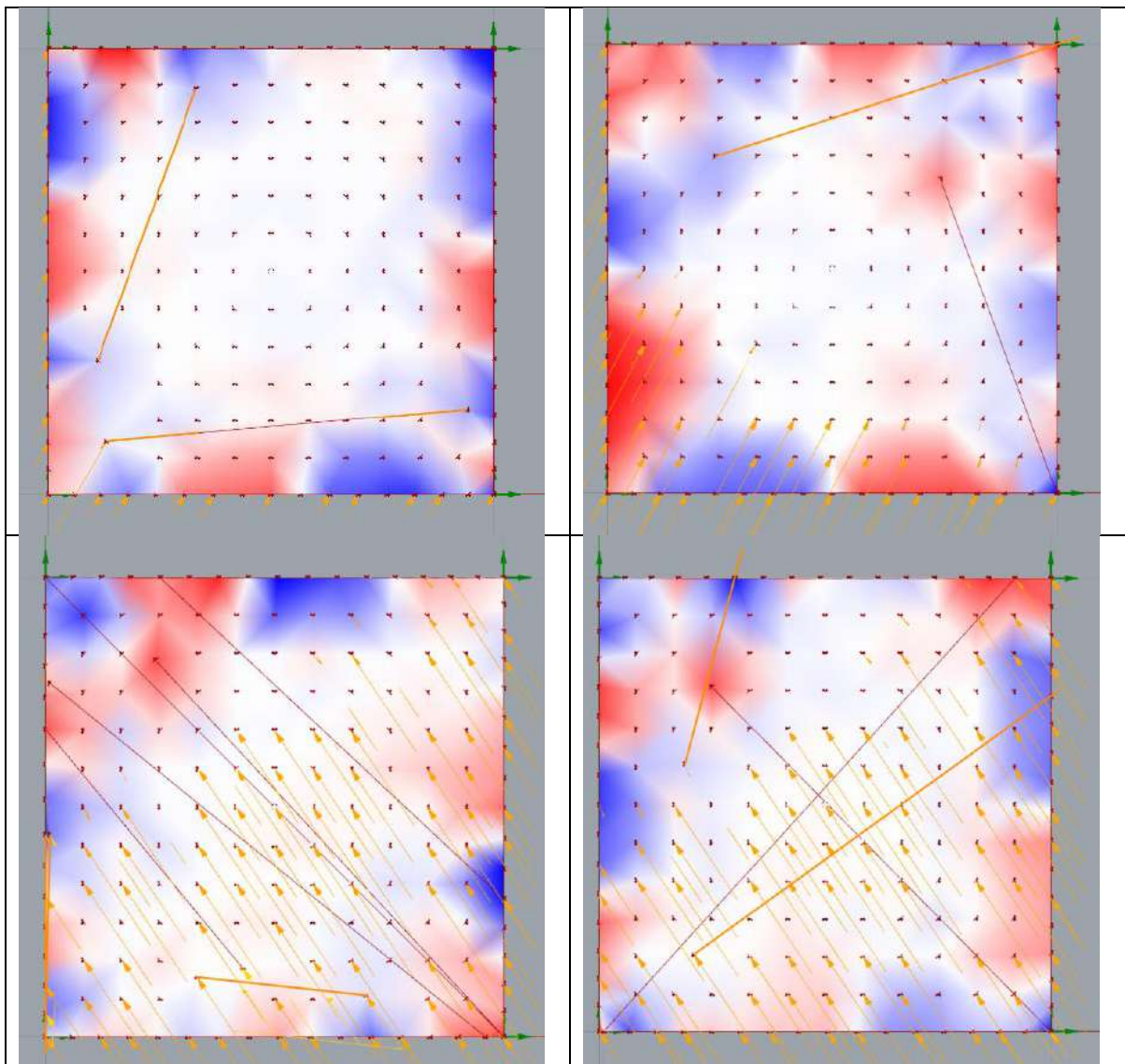
Grafika 41. Najwyraźniejsze tendencje w postaci sprężeń krawędzi powłoki oraz układów równoległych i prostopadłych. Dla dowolnego przypadku obciążeniowego model uzyskiwał jeden z wymienionych układów.
