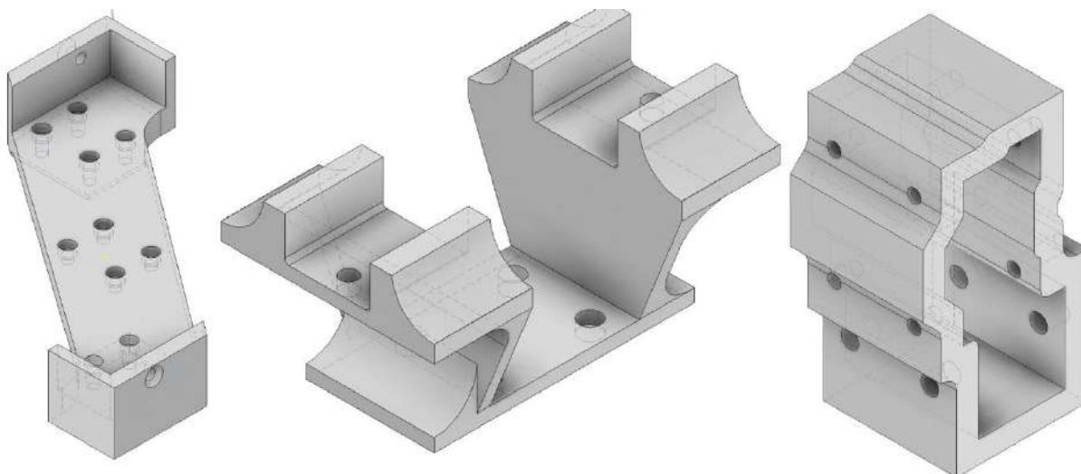
Grafika 15. Aksonometryczne prezentacje elementów podpory wykonane przez autora w programie Autodesk Inventor 2024 stanowią część załącznika nr 5.B pracy. Elementy przygotowano w module systemu v-slot 2020.
