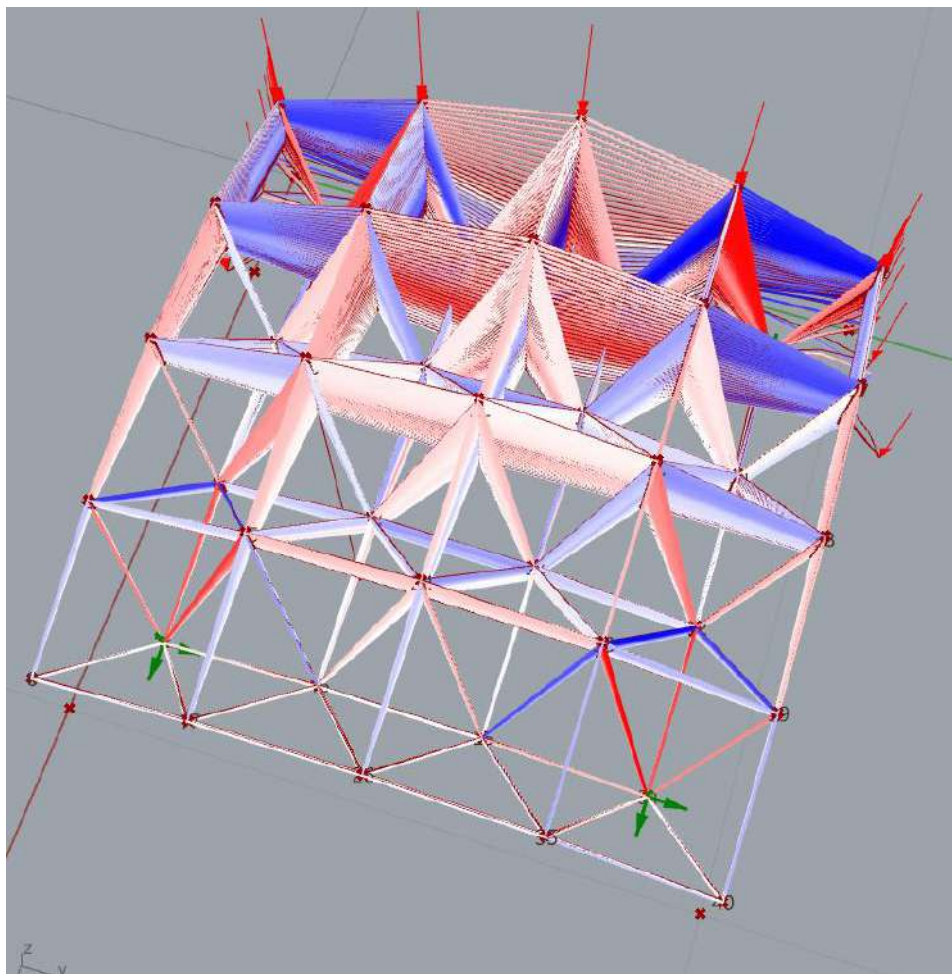
Grafika 63. Zestawienie wyników geometrycznych reakcji modelu na jeden z przypadków obciążeniowych wraz z graficzną reprezentacją naprężeń policzonych z użyciem MES.
