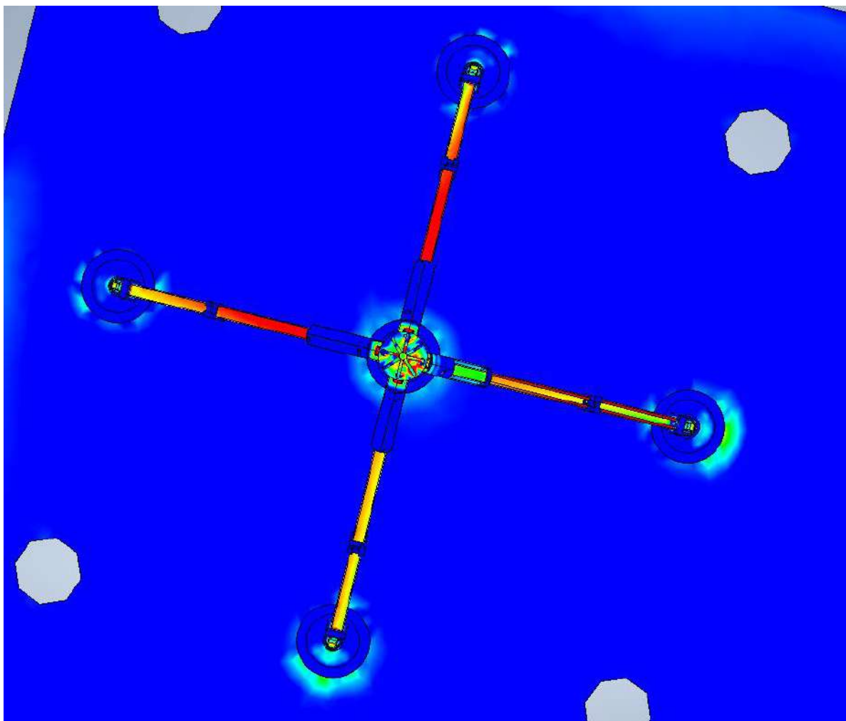
Grafika 36. Analiza MES wykonana na pojedynczym modelu modyfikatora przedstawia niejednorodność naprężeń na powierzchni siłowników. Analiza przeprowadzona z wykorzystaniem oprogramowania Autodesk Inventor Nastran.
