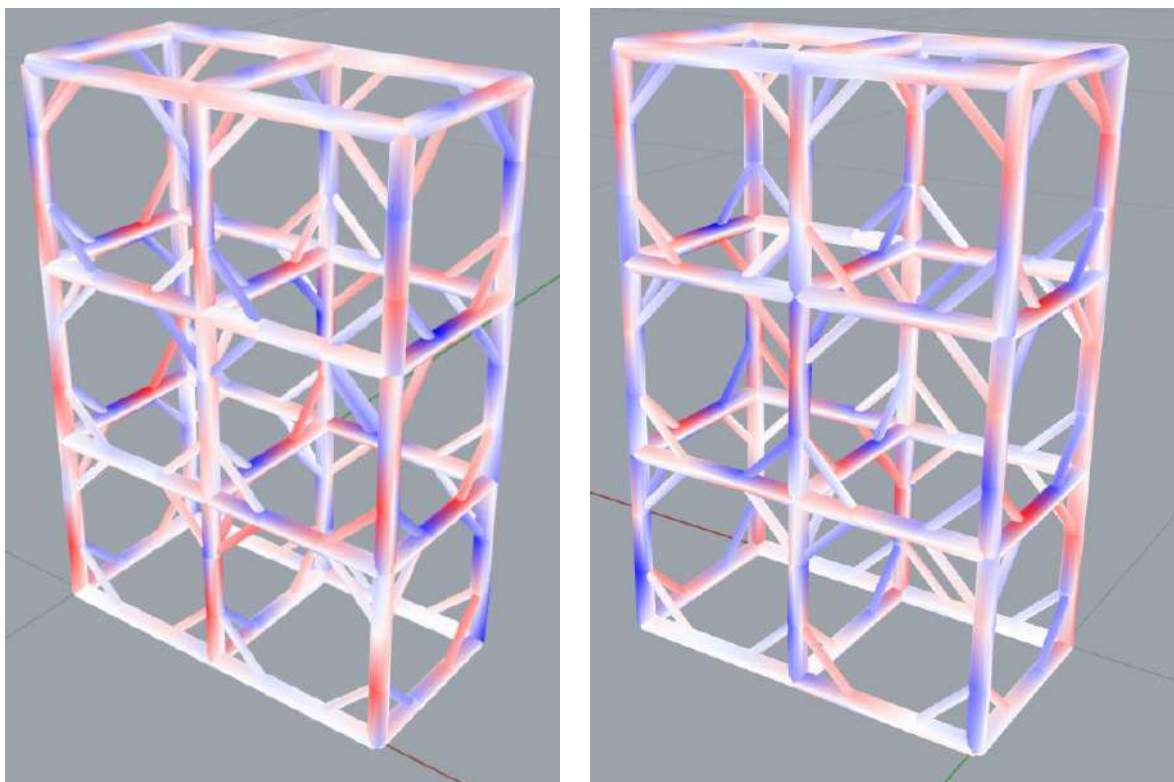
Grafika 49. Model badawczy z graficzną prezentacją wyników badań odkształceń podczas kontroli geometrii dla jednego z przypadków obciążeń poziomych zewnętrznych.
