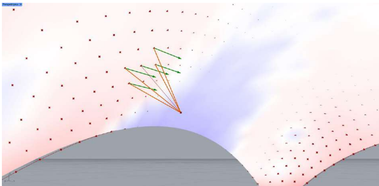
Grafika 31. Perspektywiczne zobrazowanie symulowanego modyfikatora punktowego zamocowanego w 5 punktach do powłoki. Przedstawiono uproszczenia geometryczne odpowiadające złożoności obliczeniowej modelu. Model stanowi załącznik nr 6.G pracy.
