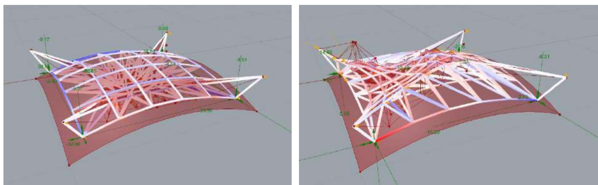
Grafika 79. Przykłady geometrii niemożliwych do uzyskania w wyniku ruchu struktury responsywnej. Model zachowań uznał układy za efektywne ze względu na brak analizy ruchów pośrednich podczas których dochodzi do szeregu niedozwolonych przecięć elementów strukturalnych.
