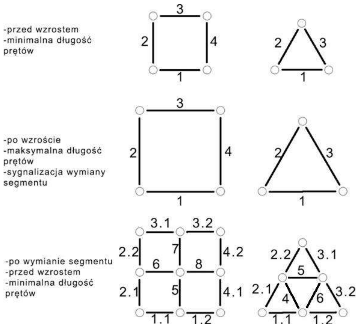
Grafika 95. Koncepcja nazewnictwa elementów struktury ekspandującej podczas wzrostu. Nazewnictwo ma na celu określenie sposobu nadzoru nad wzrostem i redukcją struktury.
