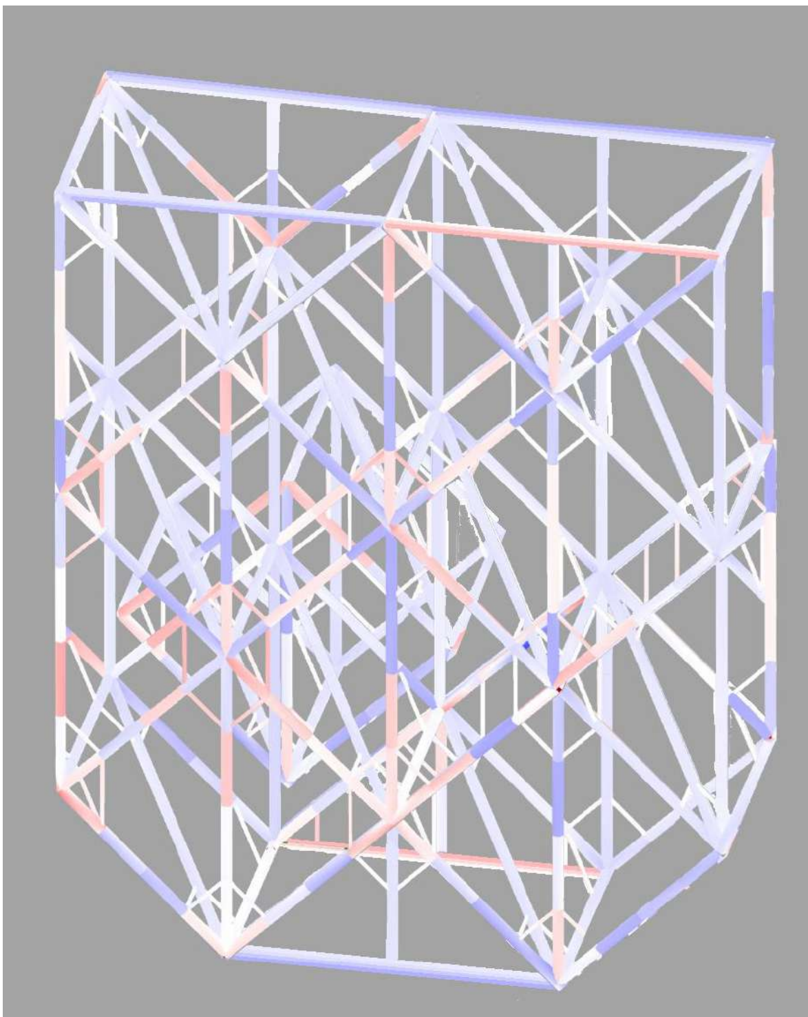
Grafika 51. Wynikowa mapa naprężeń dla struktury sztywnej topologicznie.
