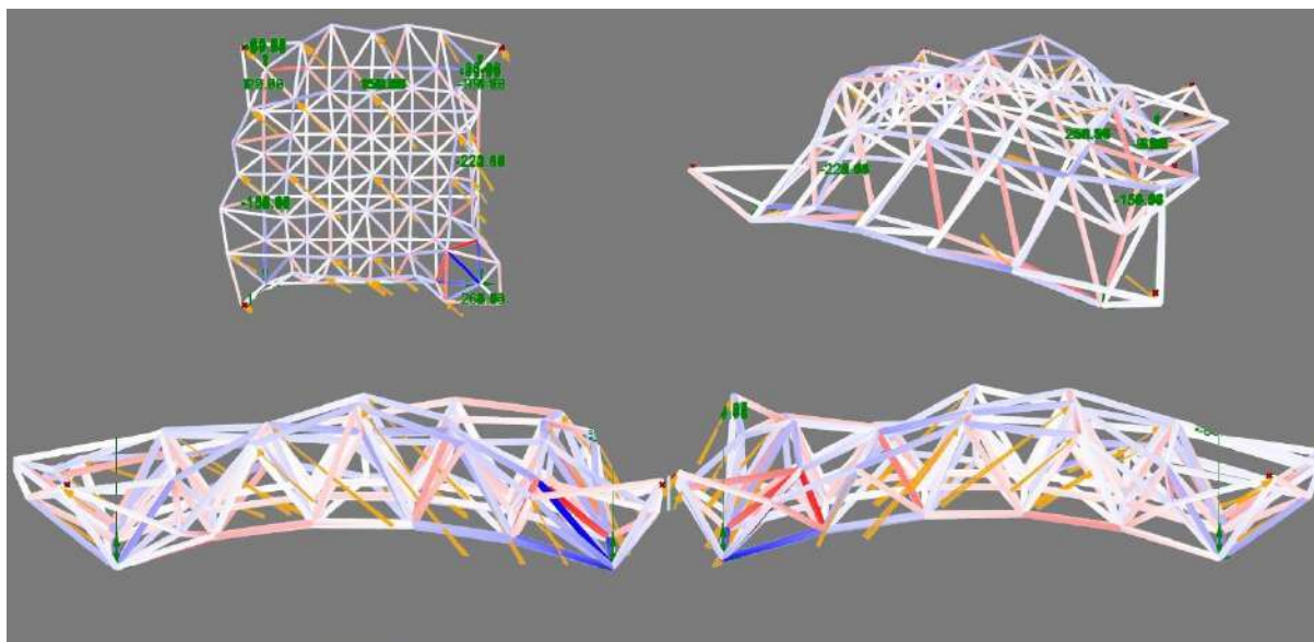
Grafika 77. Geometria struktury uzyskana w wyniku przy modelu zachowań. Charakteryzuje się bardzo dużym stopniem złożoności przestrzennej, każdy węzeł zachowuje indywidualność kierunków wyprowadzenia połączeń, a cała struktura pozostaje niezwykle wrażliwa na niedokładności wykonawcze.
