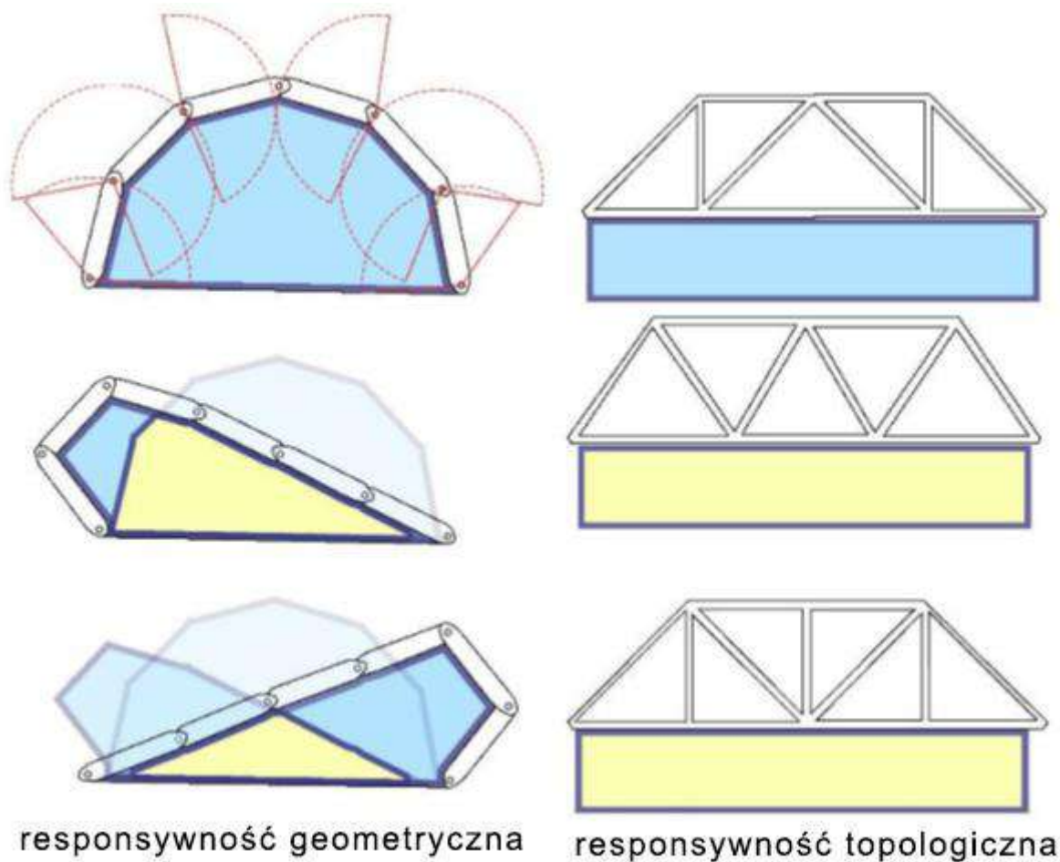
Grafika 98. Porównanie sposobu działania modeli responsywnych geometrycznie oraz topologicznie. Zauważalne jest znacznie łatwiejsze wykorzystanie responsywności topologicznej ze względu na wykorzystanie przestrzeni wokół struktury.
