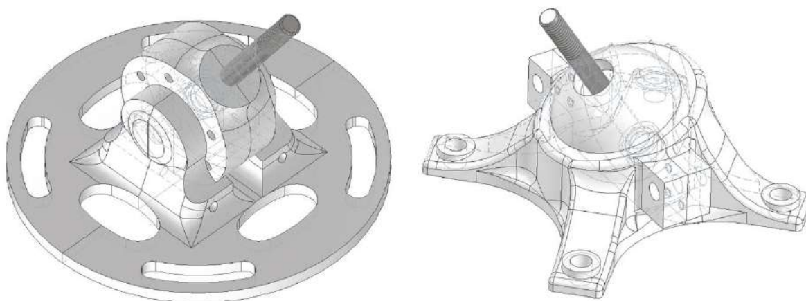
Grafika 16. Model podpory odpowiedzialny za swobodny obrót mocowania względem ruchomej części podpory. Modele stanowią załączniki nr 5.D.1 oraz 5.D.2 do pracy.
