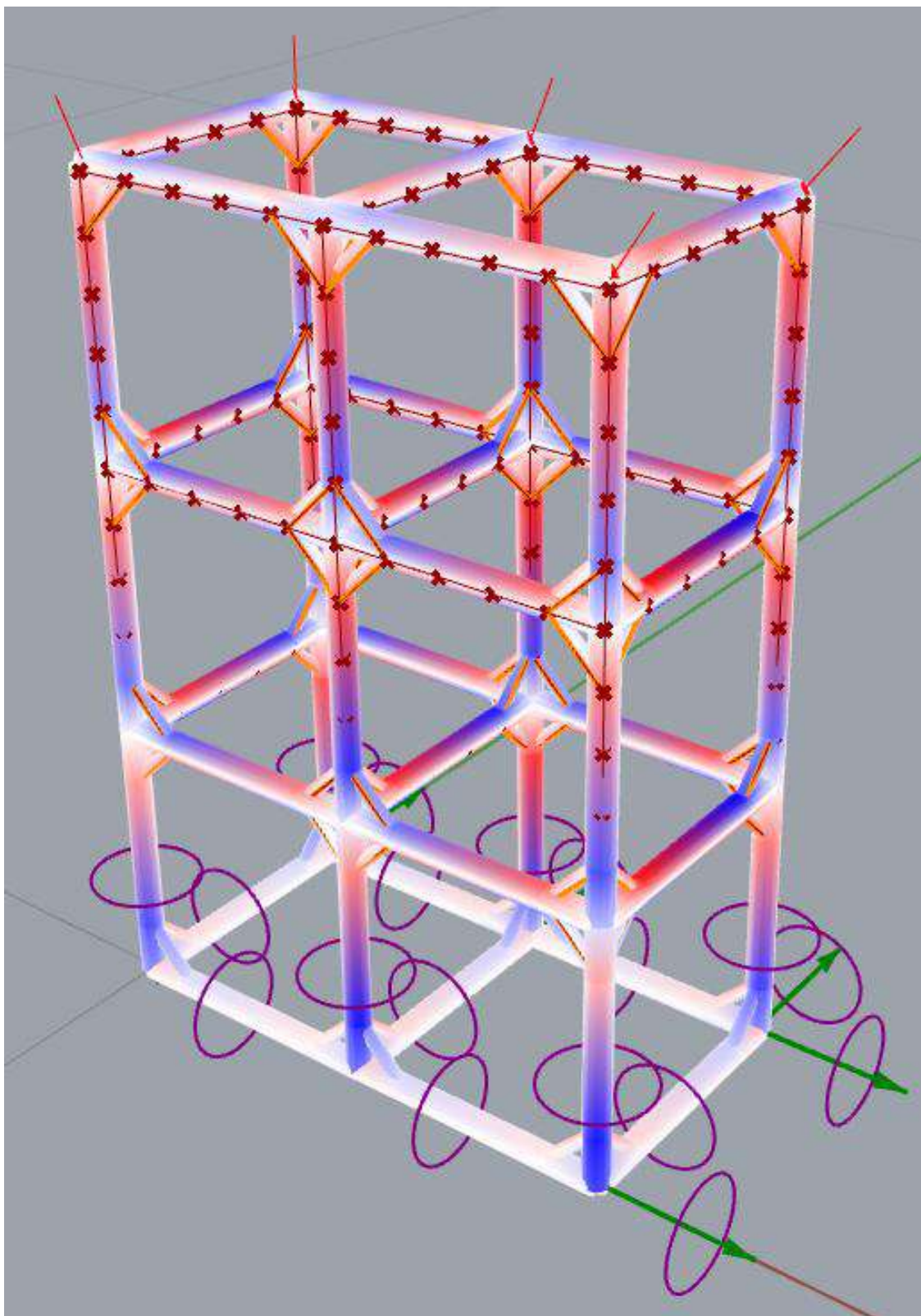
Grafika 48. Pełny model badawczy złożony z połączonych modułów elementarnych wraz z układem podpór. Model stanowi załącznik nr 7.F pracy.
