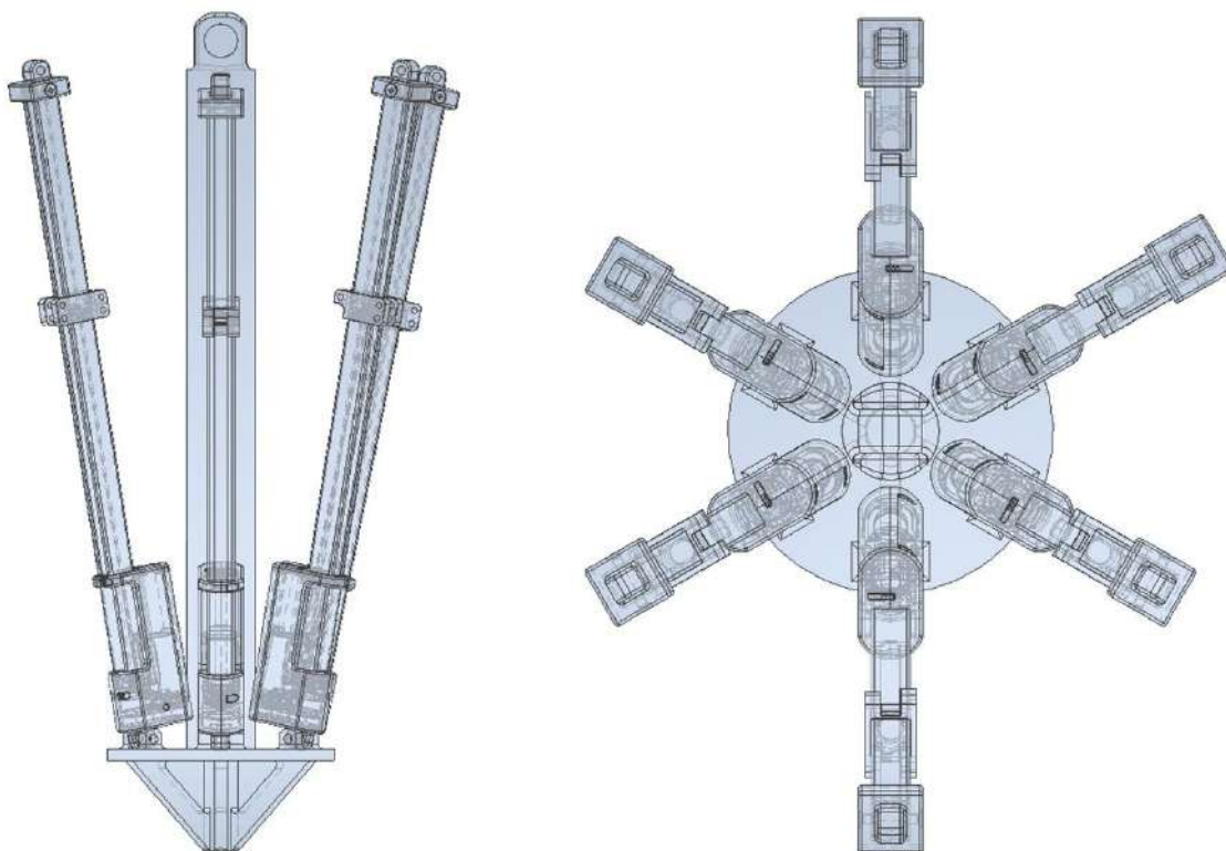
Grafika 33. Model modyfikatora wraz z 6 siłownikami oraz rdzeniem centralnym. Model opracowany w programie Autodesk Inventor 2024.
