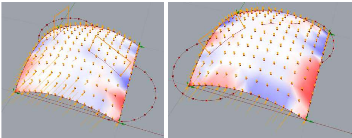
Grafika 39. Wynikowe układy modyfikatorów wraz z rozkładem naprężeń na powierzchni powłoki.
