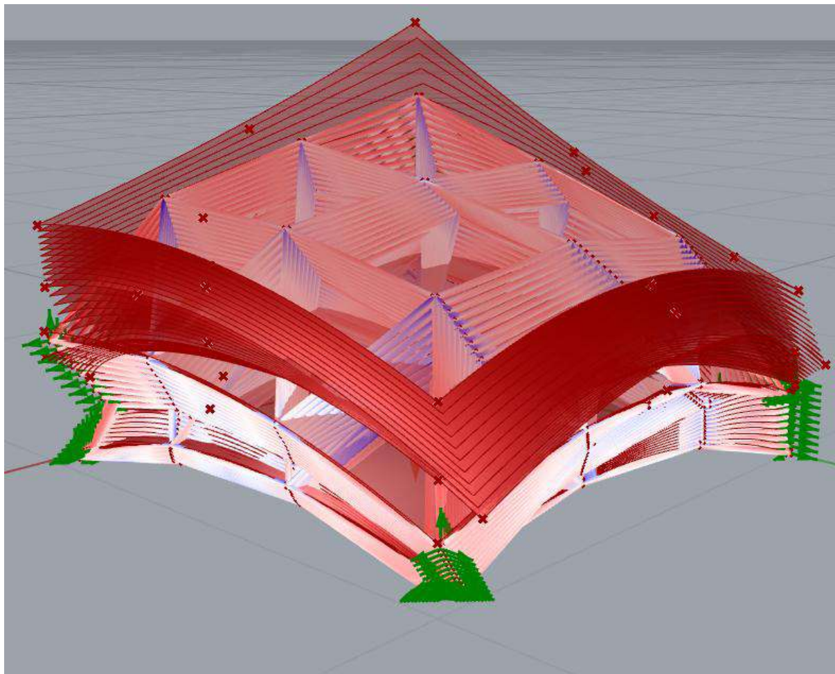
Grafika 75. Wynikowe trasowanie zmian geometrii modelu uwzględniające redukcję naprężeń w stanach pośrednich. Charakteryzuje się znacznie bardziej złożoną trajektorią translacji węzłów, lecz pozostaje opłacalna ze względu na naprężenia maksymalne.
