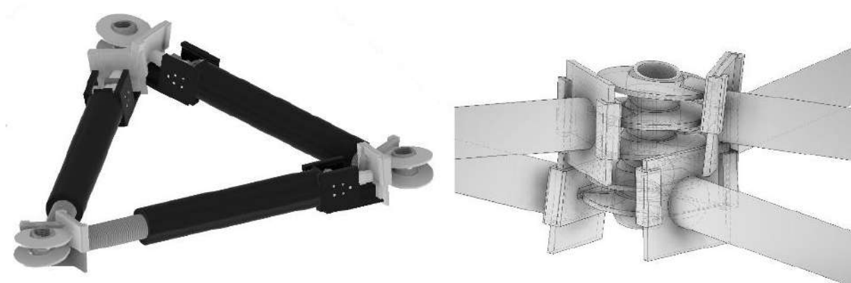
Grafika 93. Model samoformującego węzła o znacznej nieosiowości. Model nie jest limitowany liczbą połączeń wokół pojedynczego węzła.
