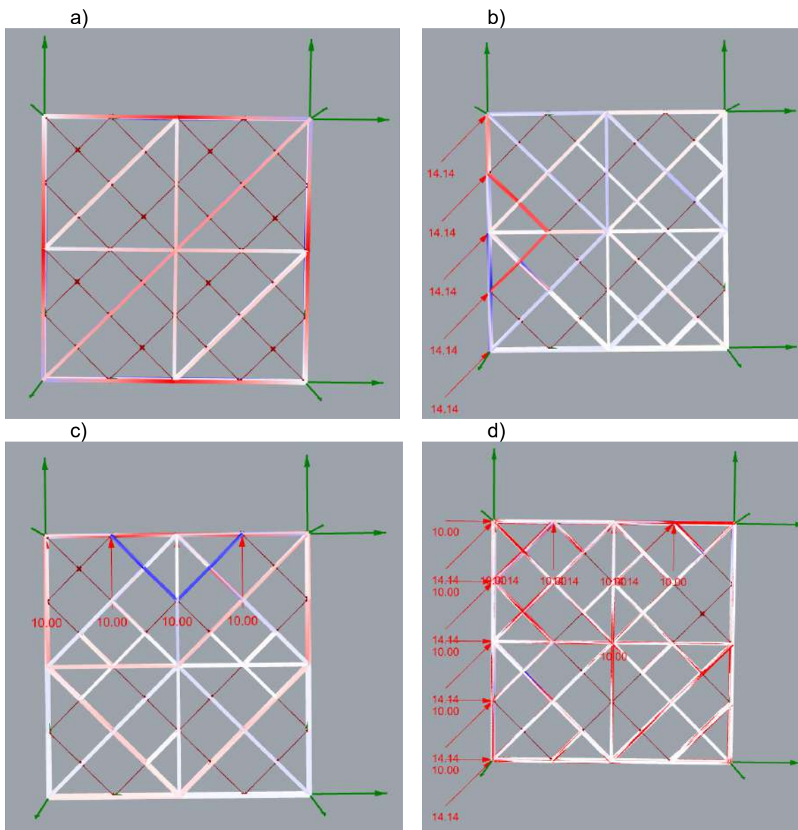
Grafika 116. Zestawienie wynikowych topologii dla wybranych przypadków badań efektywności modułów. Grafika „a)” prezentuje model sztywny nieoptymalizowany z prostym pojedynczym stężeniem ukośnym. „b)” oraz „c)” prezentują wyniki badań dla struktury responsywnej gdzie każdorazowo topologia dostosowywana jest do indywidualnego przypadku obciążeniowego. W „d)” przedstawiono efektywną topologię niezmienną dostosowaną jednocześnie do wszystkich 6 przypadków obciążeniowych.
