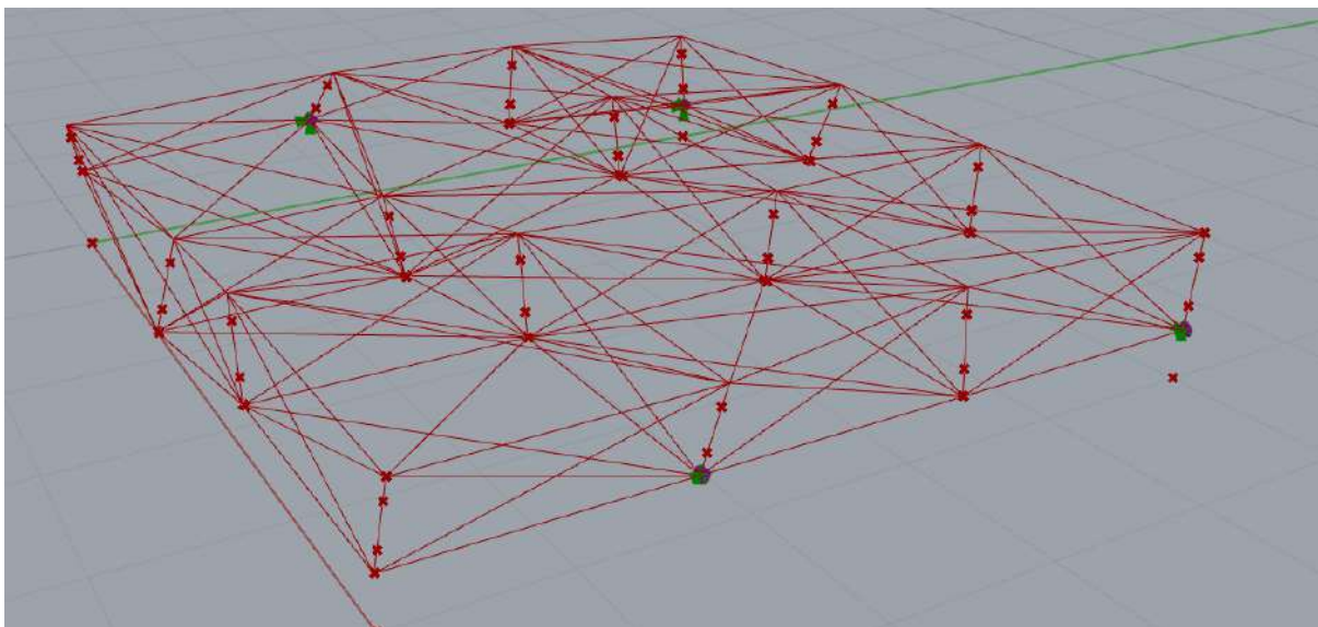
Grafika 54. Schemat liniowy struktury o swobodnej geometrii. Model posiada powtarzalne węzły pod względem topologicznym, lecz o indywidualnych zależnościach kątowych między elementami.
