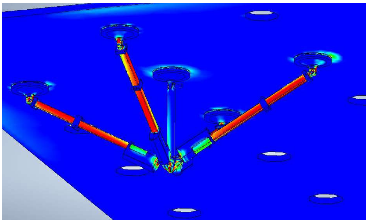
Grafika 37. Aksonometryczny widok wyników graficznych analizy MES. Strefy wokół punktów mocowania modyfikatora do powłoki charakteryzują się niskimi naprężeniami.
