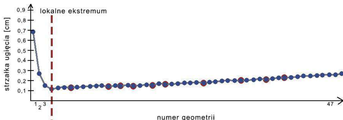
Grafika 64. Wykres zależności wartości strzałki ugięcia od stopnia intensywności reakcji modelu. Zauważalne jest jedno wyraźne ekstremum globalne oraz szereg ekstremów lokalnych wpływających na trudność uzyskiwania najefektywniejszych wyników poszukiwania geometrii z użyciem algorytmu ewolucyjnego.
