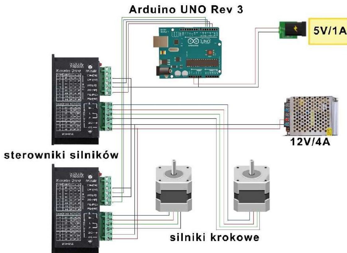
Grafika 17. Schemat elektroniki sterowania ruchem podpory z użyciem mikrokontrolera Arduino Uno Rev3 z użyciem własnego oprogramowania.
