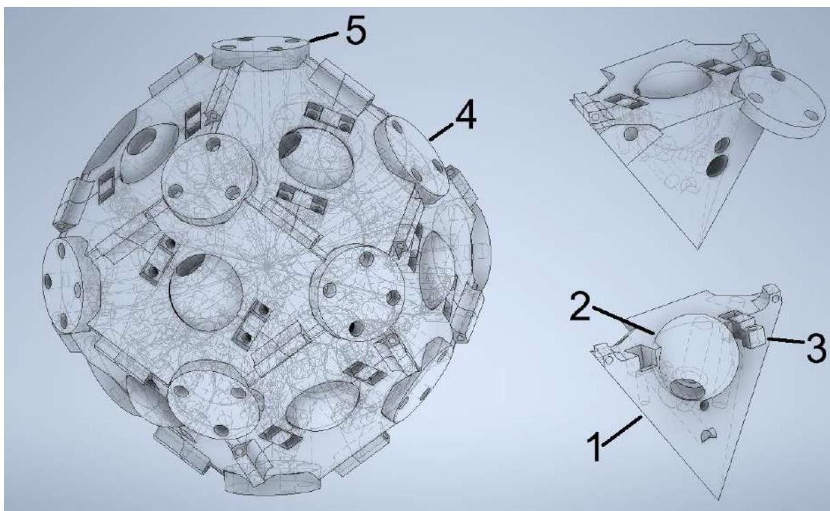
Grafika 86. Koncepcja modelu bryłowego węzła z przedstawieniem podziału na elementy złożenia. Struktura składa się z powtarzalnych 12 segmentów łączonych między sobą wielopunktowo. Węzeł uzyskuje wytrzymałość dopiero po złożeniu całości jego modelu.
