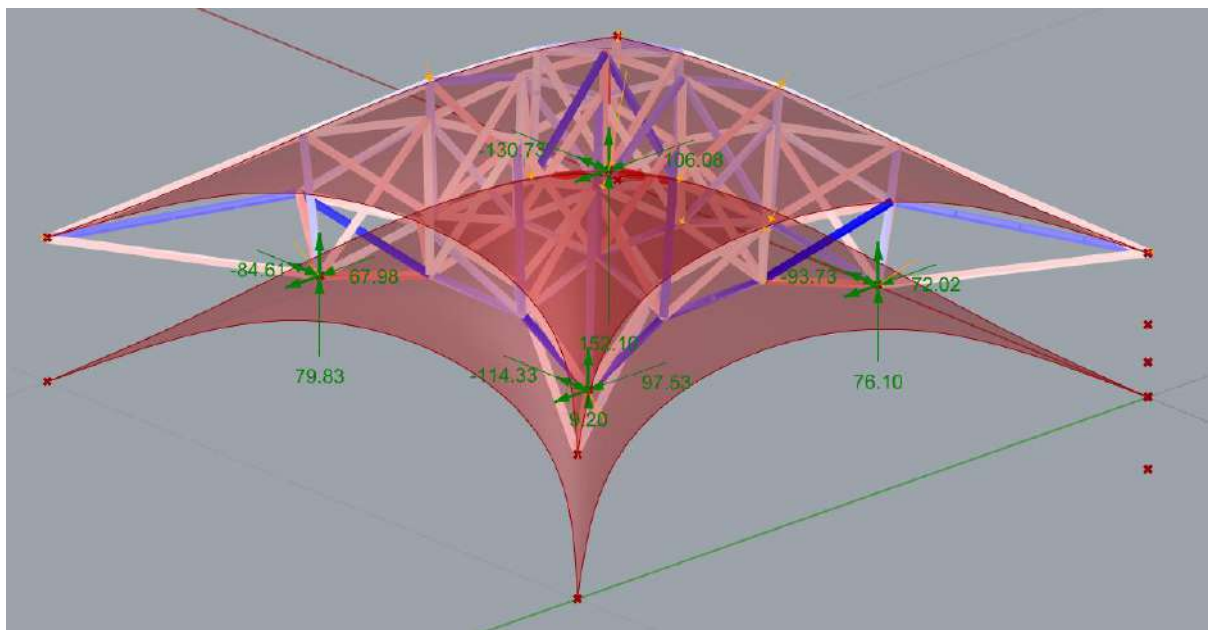
Grafika 58. Model uzyskany w wyniku działania algorytmu dynamicznych relaksacji. Model stanowi załącznik nr 8.E pracy.
