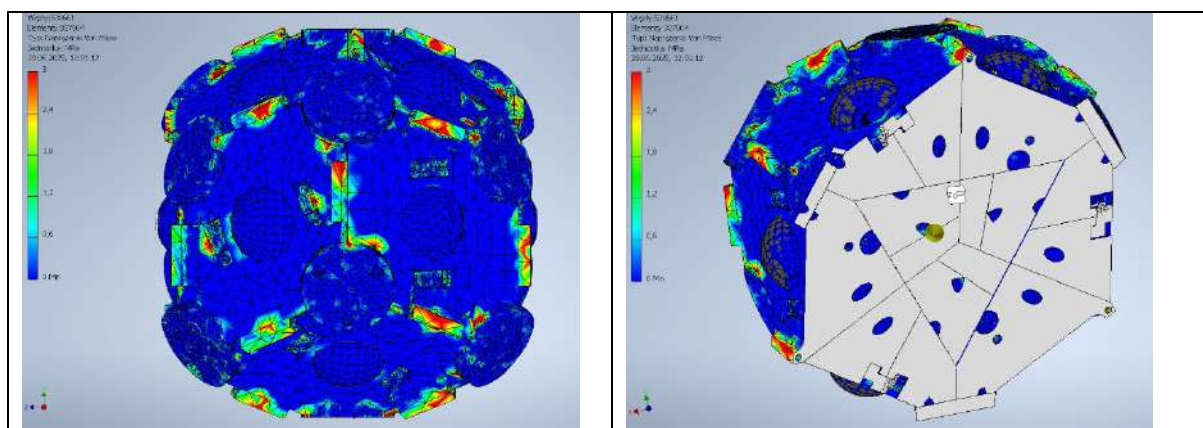
Grafika 87. Wyniki analizy MES rozkładu naprężeń w strukturze obciążonej siłami osiowymi 3 prętów wywołujących obrót modelu. Na prawej grafice widoczny jest przekrój przez węzeł prezentujący podział na elementy składowe modelu.
