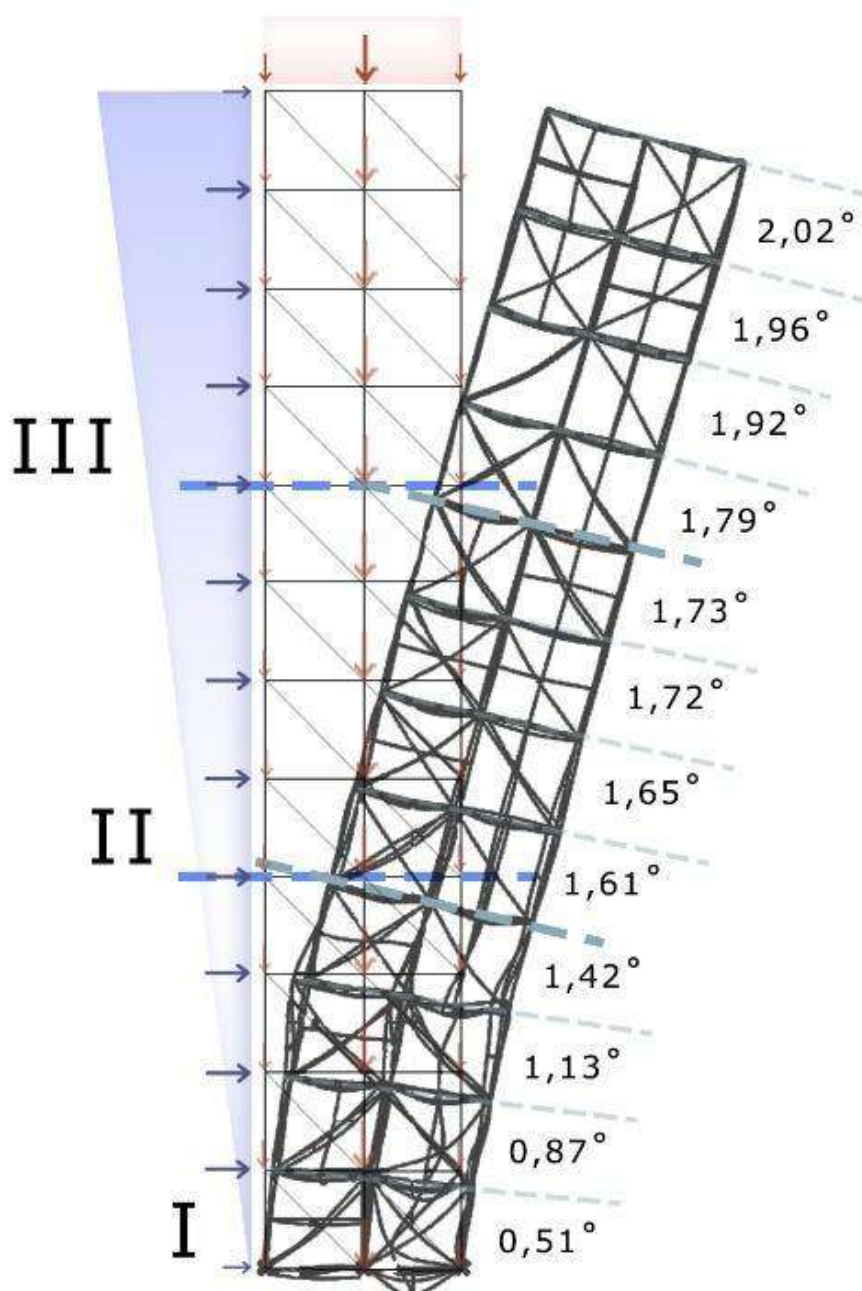
Grafika 102. Geometria zdeformowanej obciążeniami struktury. Odchylenie od pionu liczone jest dla poziomych pasm prętów każdego poziomu modułów osobno.
