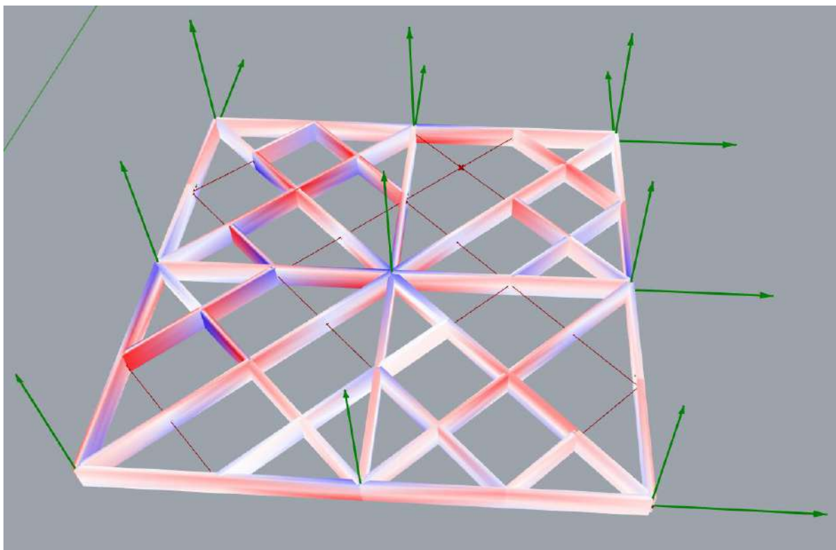
Grafika 115. Przygotowany model symulacji zachowań 4 modułów złożonych z 8 półmodułów. układ wsparty na 4 narożach poddawany jest obciążeniom w każdej płaszczyźnie, a wynik w czasie rzeczywistym prezentowane są w formie graficznych wykresów na modelu.
