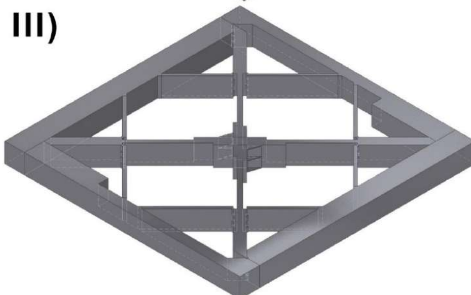
Grafika 111. Przedstawienie modelu modułu responsywnego topologicznie w 3 kolejnych fazach rozkładania. Model opracowano przy użyciu oprogramowania Autodesk Inventor Professional 2024 i stanowi załącznik do pracy.
