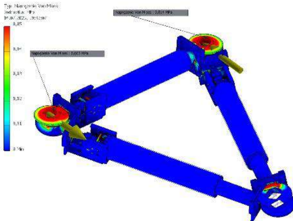
Grafika 94. Wynik analizy MES modelu trzelementowej struktury samoekspandującej. Główne naprężenia zgodnie z wykresem zlokalizowane są w otoczeniu węzłów.
