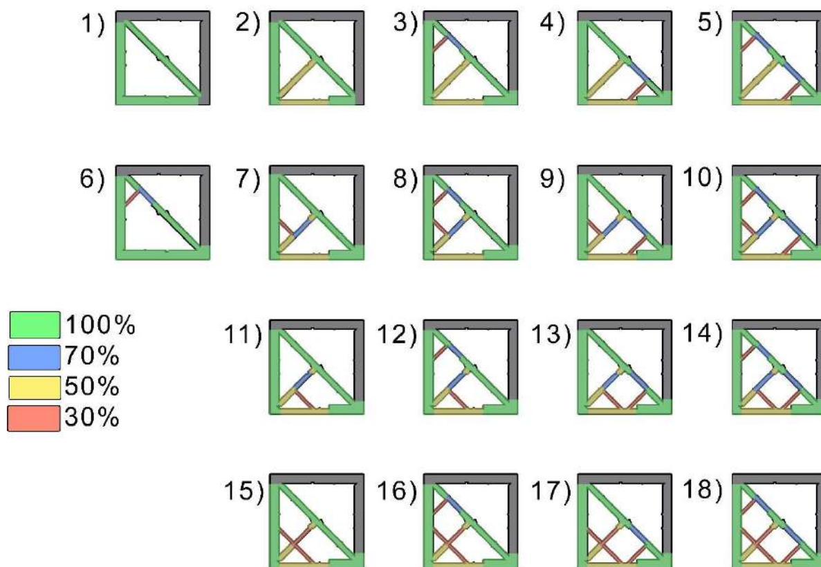
Grafika 113. Matryca przypadków sztywności modułu przygotowana na cele programowania zachowań struktury podczas symulacji. Procenty odnoszą się do szerokości przekroju względem wartości referencyjnej 20cm. Parametr ten bezpośrednio wpływa na momenty bezwładności oraz dalej wytrzymałość modułu.
