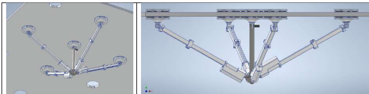
Grafika 34. Model siłownika 5-punktowego połączonego z powłoką. Przedstawiono sposób wykorzystania łączników rozkładających naprężenia. Model opracowano w programie Autodesk Inventor Professional 2024 i stanowi załącznik nr 6.E pracy.
