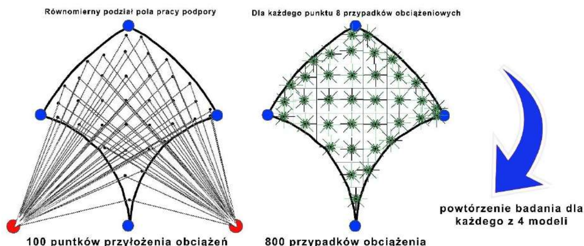
Grafika 26. Schemat układu obciążeń na cele badania jednolitości rozkładu naprężeń.
