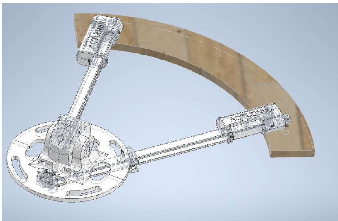
Grafika 21. Model podpory opartej na dwóch siłownikach. Sterowanie odbywa się poprzez ruch biegunowy dwóch siłowników. Model wykonano przy użyciu programu Autodesk Inventor Professional 2024. Stanowi on załącznik nr 5.C pracy.
