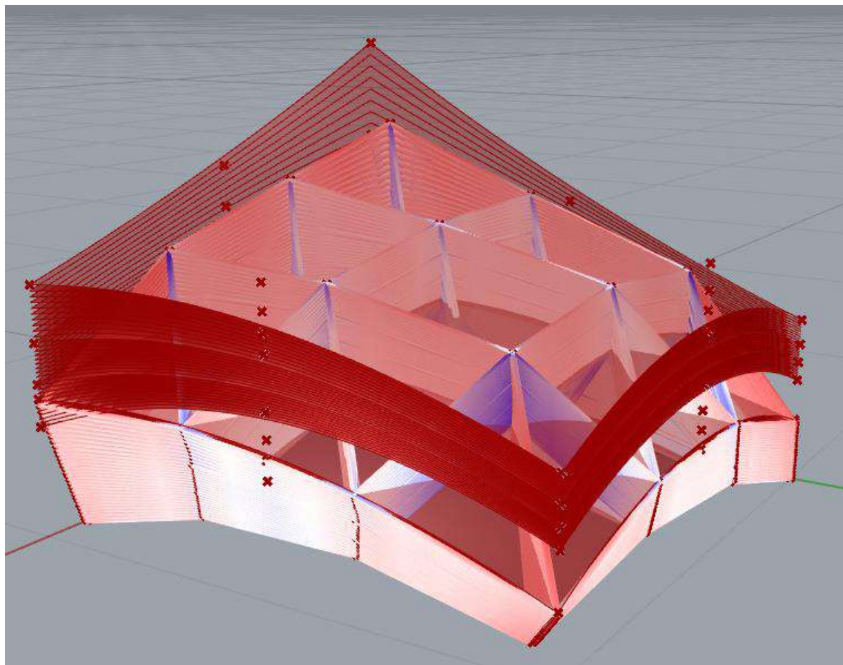
Grafika 73. Model badawczy ruchów pośrednich z płaszczyznami na których rozciągnięta jest kratownica przestrzenna. Zaznaczone są widoczne punkty geometrii pośrednich sterowanych algorytmem ewolucyjnym.
