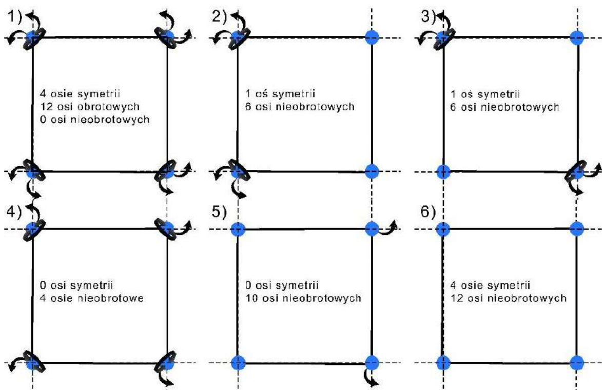
Grafika 12. Schemat układu typów podpór w strukturze. Dla każdego układu powłoka wsparta jest w 4 punktach narożnych, lecz zawsze zróżnicowany pozostaje układ stopni swobody.
