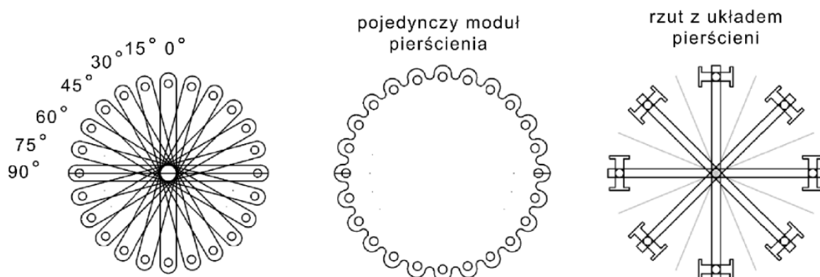
Grafika 81. Koncepcyjne opracowanie budowy węzła w drugiej płaszczyźnie ze względu na dostępność do punktów połączeń węzła z prętami.
