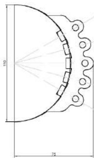
moduł ukośny 5-gniazdowy
