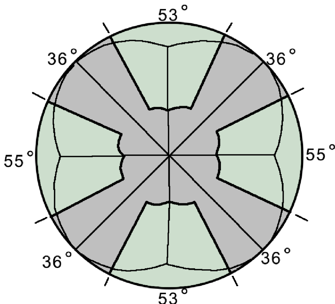
Grafika 91. Schemat zakresów ruchu poszczególnych połączeń węzła z prętami. Kolorem zielonych przedstawiono przestrzeń ruchu pojedynczych połączeń. Kolorem szarym zaznaczono martwą strefę węzła służącą równomiernej dystrybucji naprężeń w bryle węzła.
