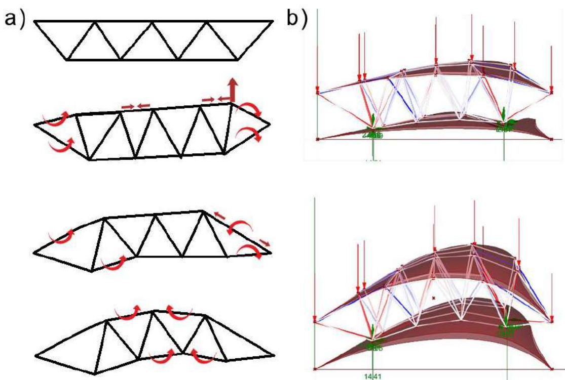
Grafika 70. "a)" przykład modelu stosującego sekwencjonowanie ruchu podczas zmiany geometrii. "b)" zmiana geometrii modelu podczas prostej transformacji między kolejnymi geometriami. Model sekwencyjowany uzyskuje znaczną redukcję naprężeń podczas ruchu względem modelu referencyjnego.
