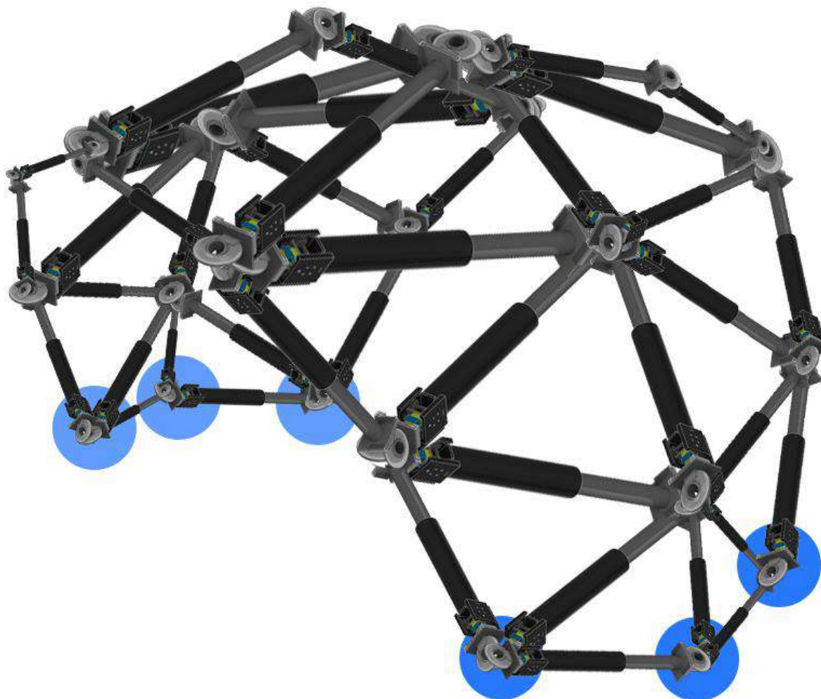
Grafika 97. Koncepcja modelu samoekspandującego struktury jednowarstwowej z elementów teleskopowanych.
