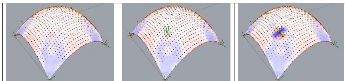
Grafika 32. etapy lokalizacji modyfikatorów na powierzchni powłoki w celu symulacji procesu aktywnego wyginania 13
