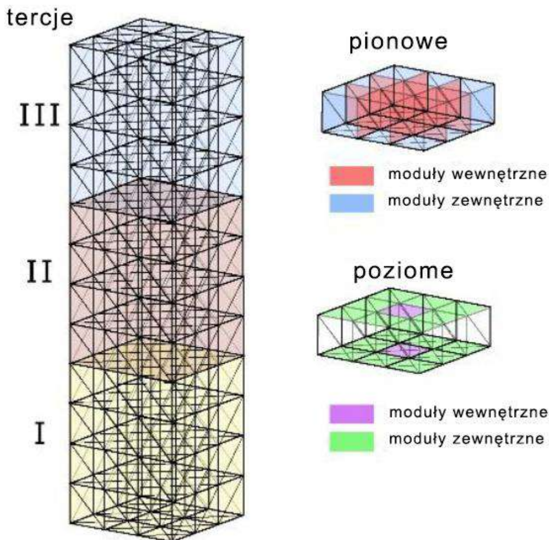
Grafika 104. Podział modelu badawczego na elementy przynależne konkretnym segmentom struktury. Na podstawie przedstawionego podziału liczono dalej istotność udziału elementów w całkowitej sztywności modelu.
