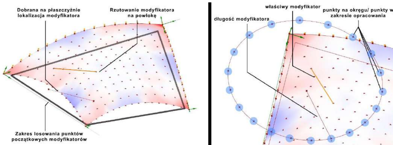
Grafika 38. Uproszczona geometryczna budowa siłownika i sposób doboru punktu mocowania drugiego końca wraz z rzutowaniem siłownika na powłokę.
