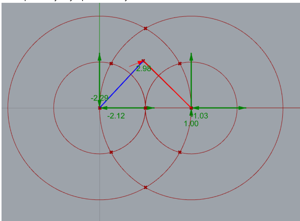
Grafika 23. Widok z góry układu podpory. Wszystkie parametry geometryczne pozostają zmienne co pozwala na proste dostosowanie zakresu ruchu modelu oraz formy jego granic. Model badania podpory został wykonany w programie Rhinoceros Grasshopper i stanowi załącznik nr 5.H pracy.
