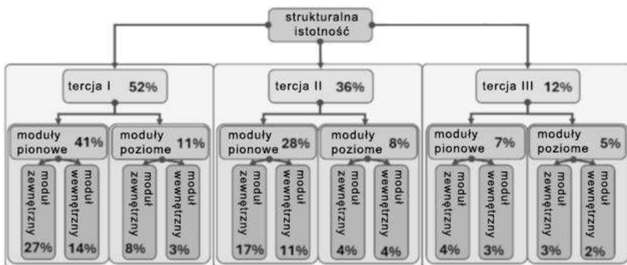
Grafika 103. Przedstawienie wyników wpływu poszczególnych elementów na sztywność całkowitą struktury. Widoczny jest największy wpływ elementów dolnej sekcji.
