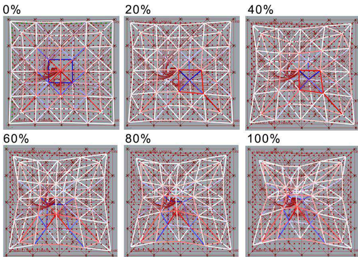
Grafika 69. Kolejne fazy zmiany geometrii struktury sterowanej modelem nr 4 między geometrią referencyjną, a docelową. Zauważalne są znaczne zmiany układu naprężeń wymagające pogłębionej analizy statycznej.
