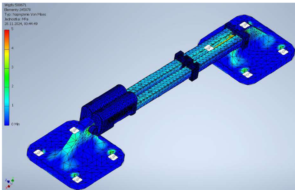
Grafika 43. Model siłownika z przedstawieniem graficznych wyników analizy MES. Model przygotowano w oprogramowaniu Autodesk Inventor Professional 2024, a następnie przebadano w Autodesk Inventor Nastran z użyciem nieliniowej analizy statycznej. Plik modelu modyfikatora stanowi załącznik nr 6.A pracy.
