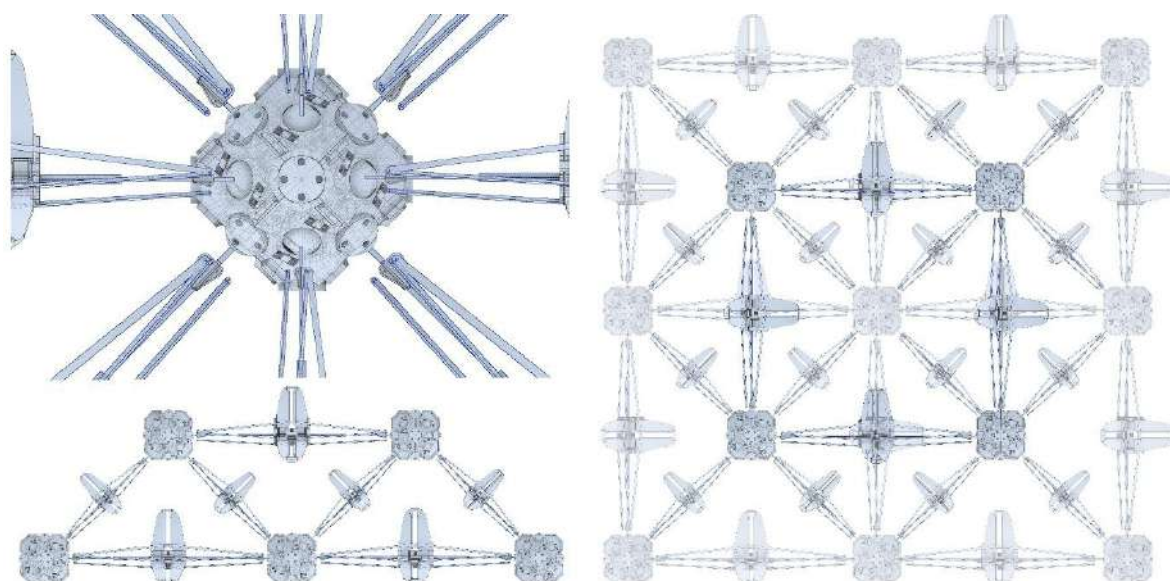
Grafika 88. Koncepcja struktury możliwa do uzyskania w wyniku użycia systemowych węzłów opracowanych w opisanych badaniach. Węzeł w szczególności predestynowany jest do użycia w strukturach o powtarzalnych modułach strukturalnych.
