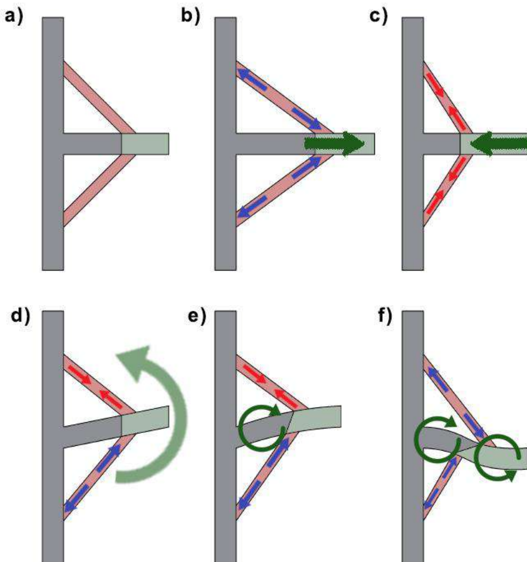
Grafika 45. Sposoby wpływu na geometrię strefy węzłowej struktury z wykorzystaniem modyfikatorów.
