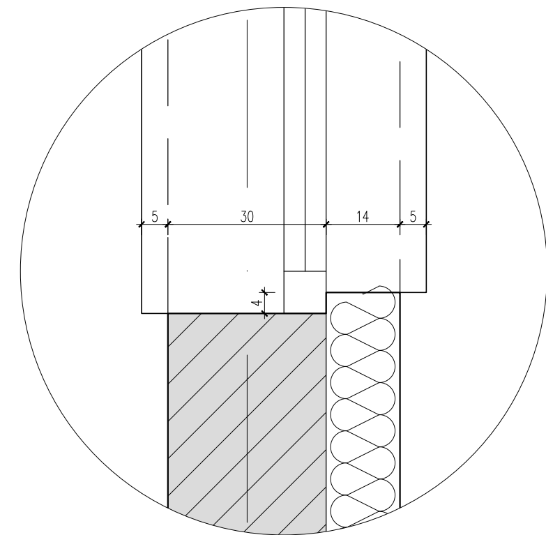
detal węgarka okiennego 1:10
