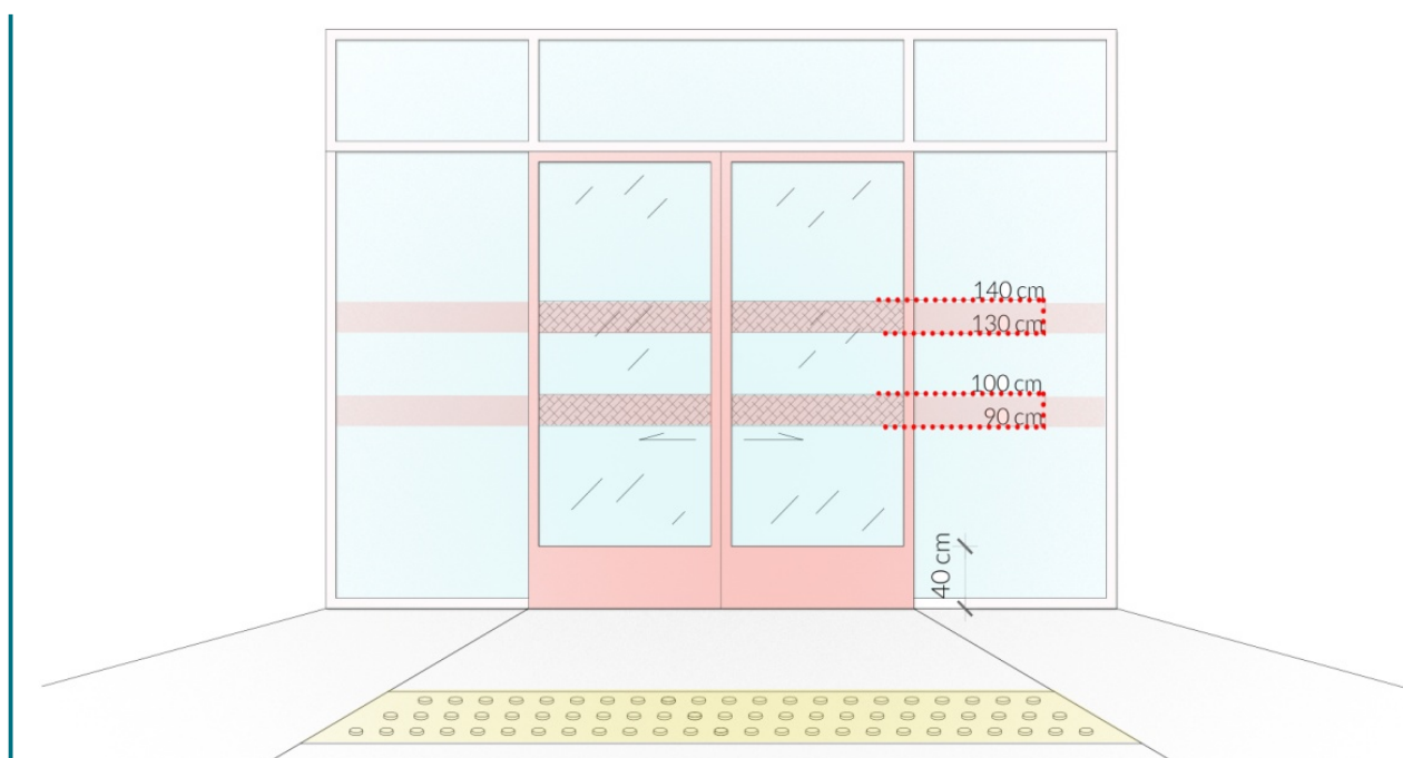
Rys. 59 Drzwi i przegrody szklane i ich oznaczenia
