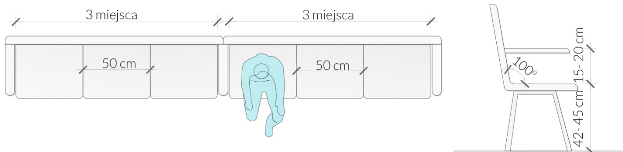
Rys. 28 Wytyczne i wymiary dotyczące ławek
